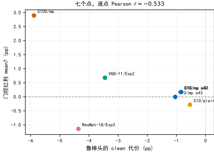
图 9: 门控红利不随鲁棒头代价单调增长。横轴为鲁棒头相对于干净头在 \alpha = 0 的精度损失（负值 = 鲁棒头更差），纵轴为门控相对单用鲁棒头在 mean7 上的增益。七个点取自四个主干配置与两个数据集，各 3 个种子。逐点 Pearson r = -0.533 ；去掉 CIFAR-100 远点后 n = 6 时符号反转为 +0.351 。数据: v5_full_recipe/recipe*.csv。
