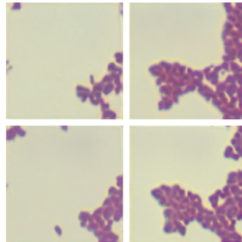
Dataset-Bacteria Diffusion-GAN
