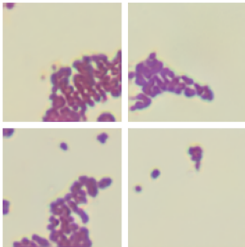
Dataset-Bacteria StyleGAN2-ADA
