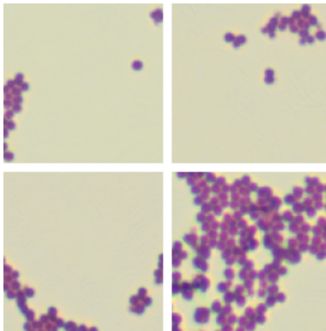
Dataset-Bacteria StyleGAN3-T
