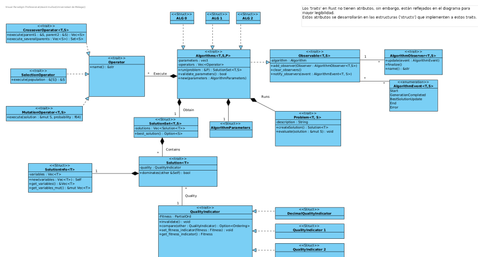
Figura 2. Arquitectura de la biblioteca. Diagrama de clases, UML. Visual Paradigm 17.0 [9].
