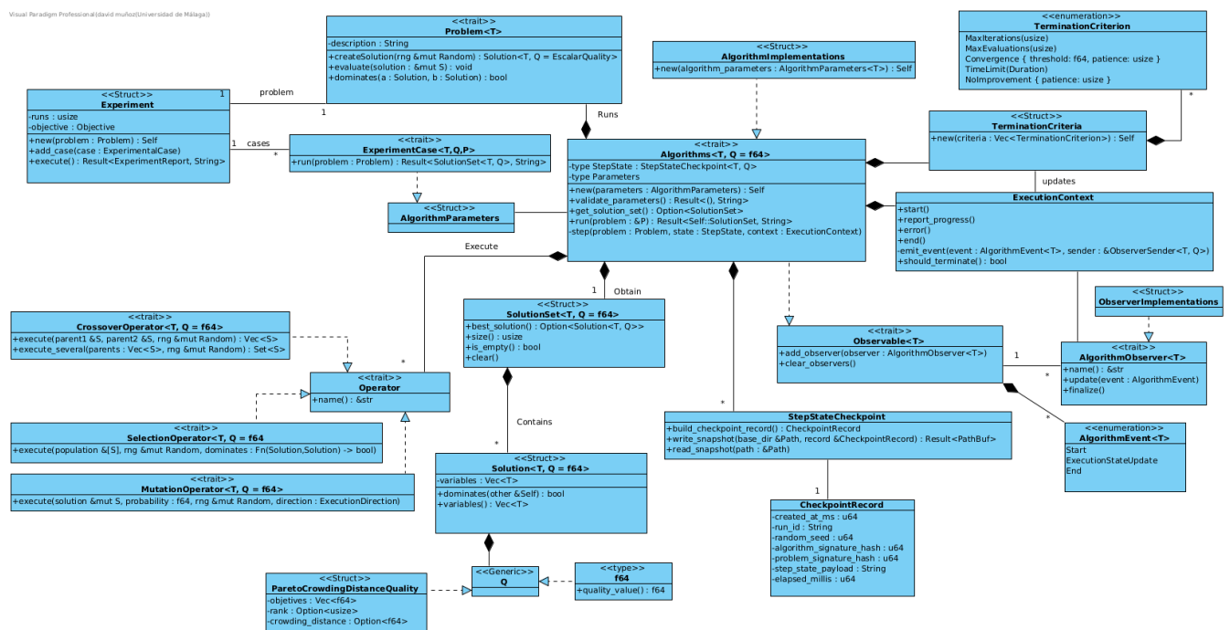
Figura 4.1. Arquitectura de la biblioteca. Diagrama de clases, UML. Visual Paradigm 17.0 [23].
