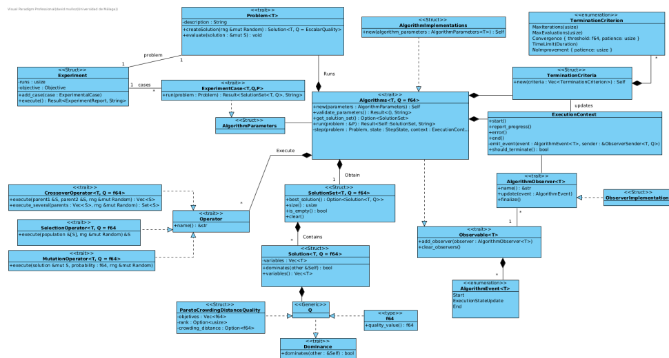
Figura 4.1. Arquitectura de la biblioteca. Diagrama de clases, UML. Visual Paradigm 17.0 [14].
