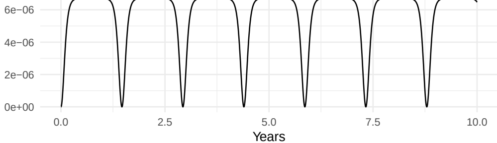
verlet
