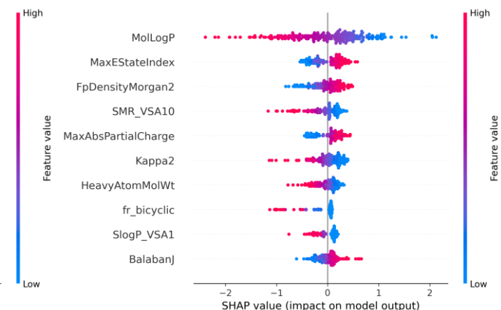
(b) ESOL
