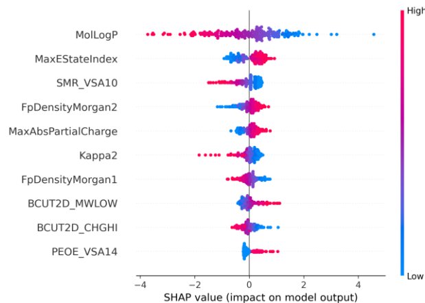
(b) ESOL
