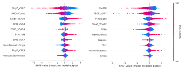
(d) Solubility
