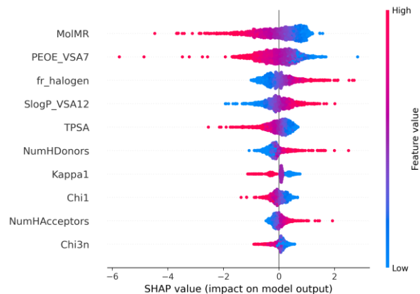
(d) Solubility, Kronecker-product
