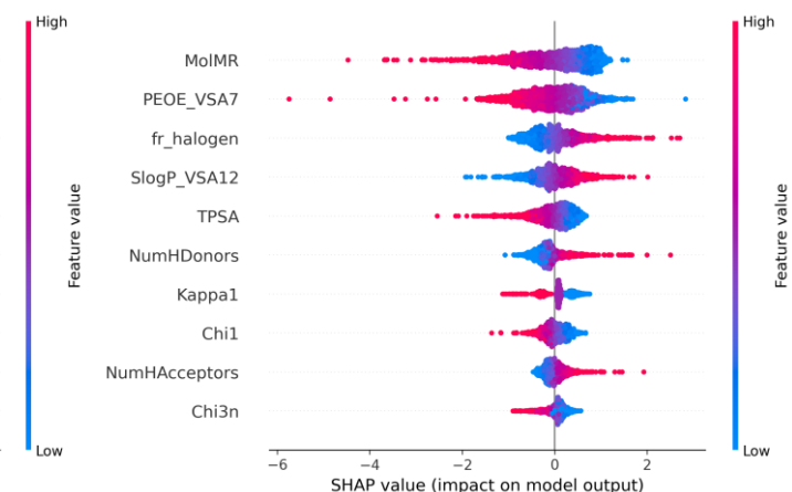
(d) Solubility
