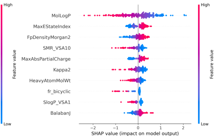
(b) ESOL
