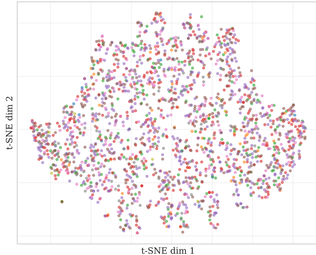
MAML
