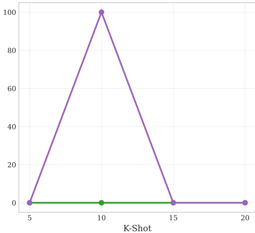
MAML
