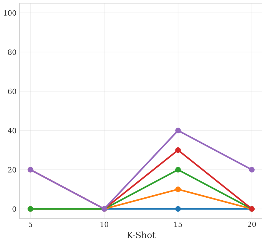
MAML
