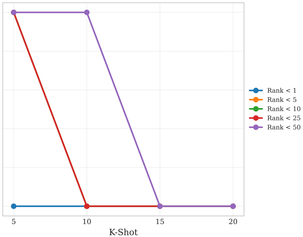
Siamese
