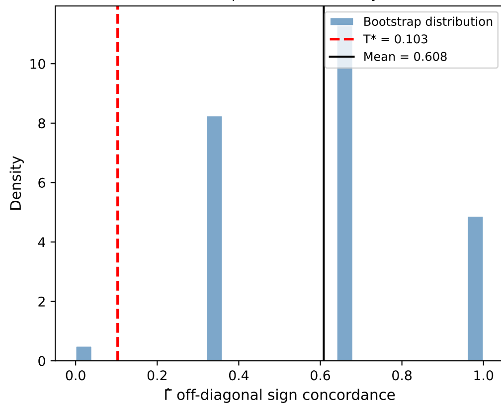
(d) Bootstrap T^* calibration (Layer A)
