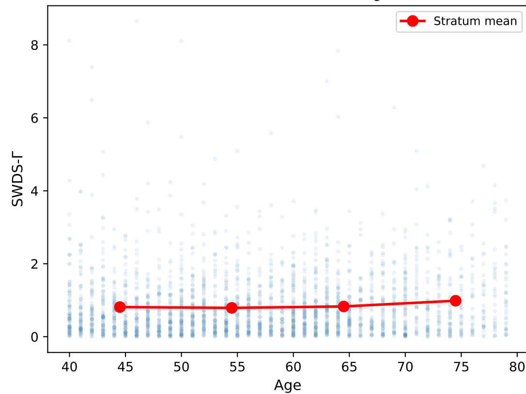
(d) Individual SWDS- \Gamma vs age
