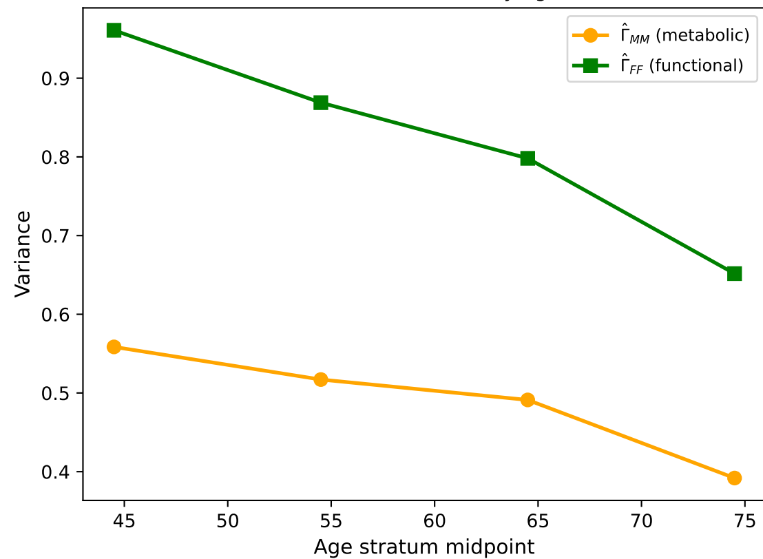
(d) Individual SWDS- \Gamma vs age
