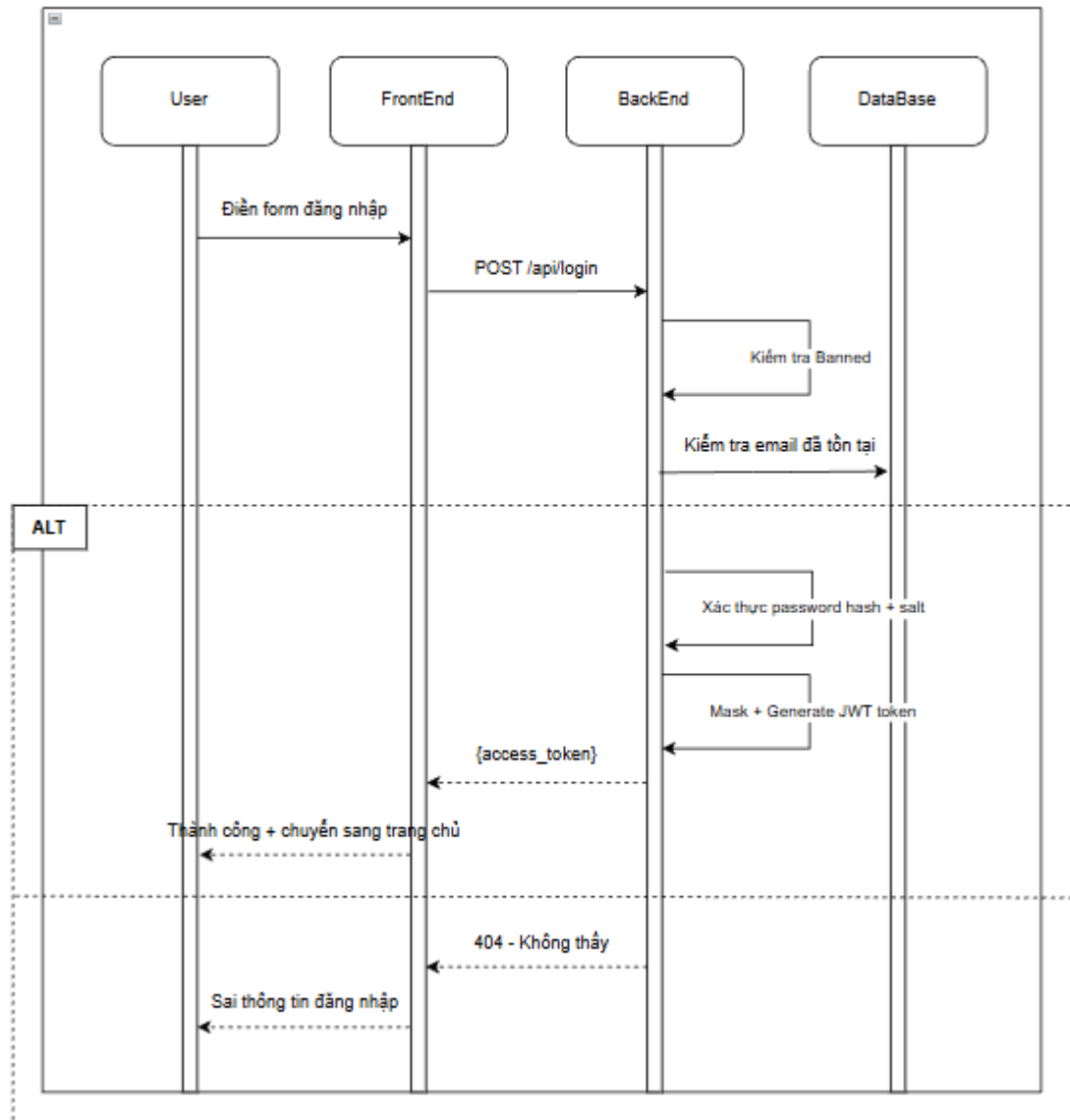
Hình 3.4 Biểu đồ tuần tự chức năng đăng nhập
