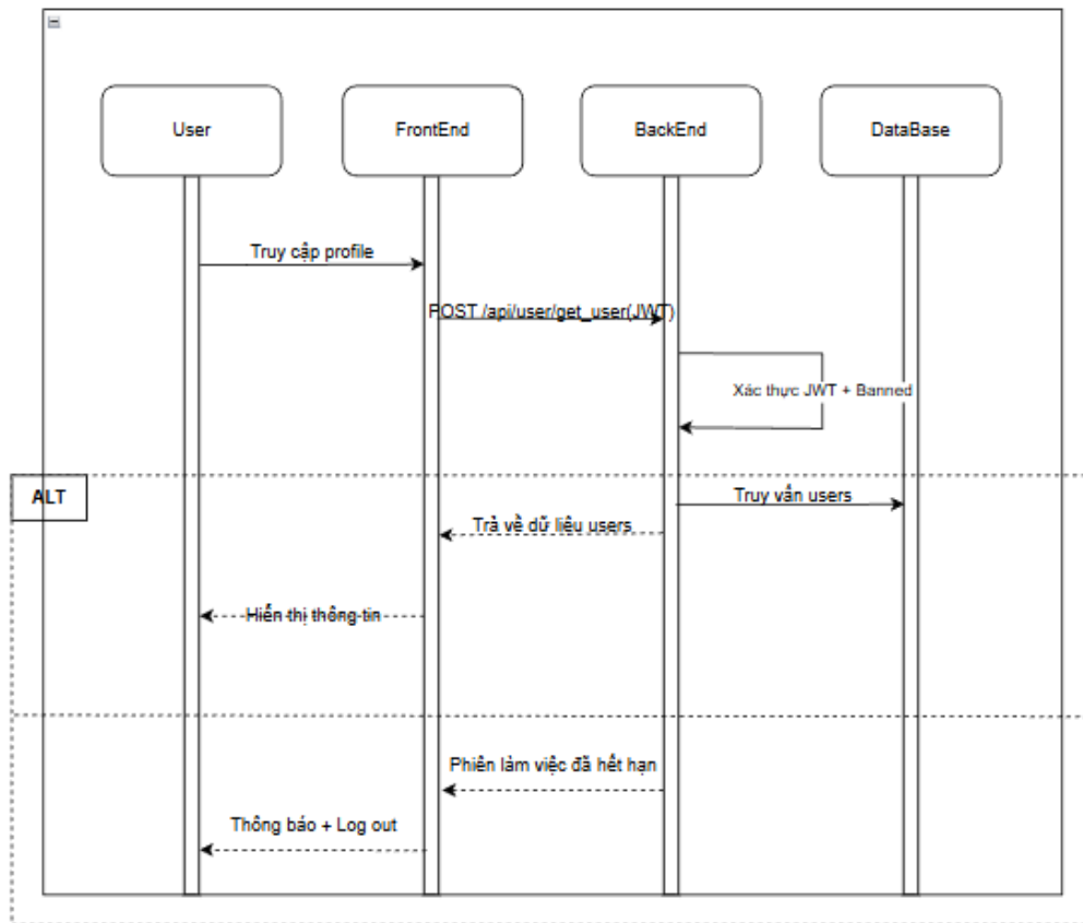
Hình 3.8 Quản lý thông tin cá nhân
