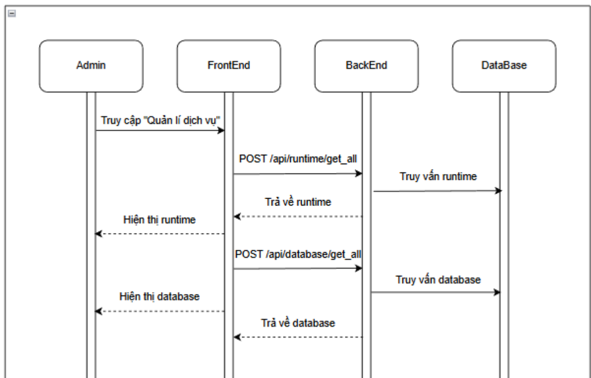
Hình 3.9 Quản lý dịch vụ
