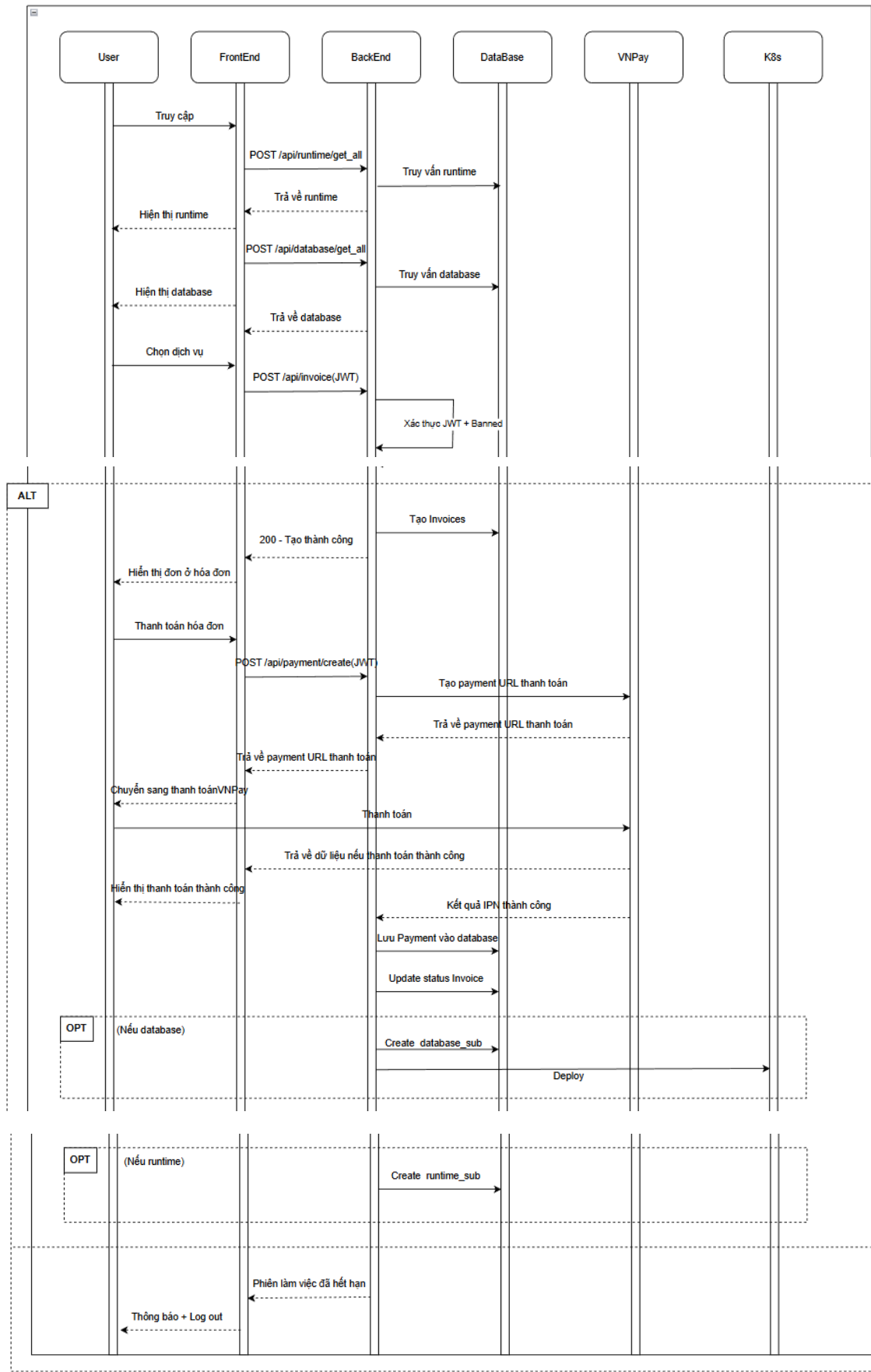
Hình 3.11 Đăng ký dịch vụ
