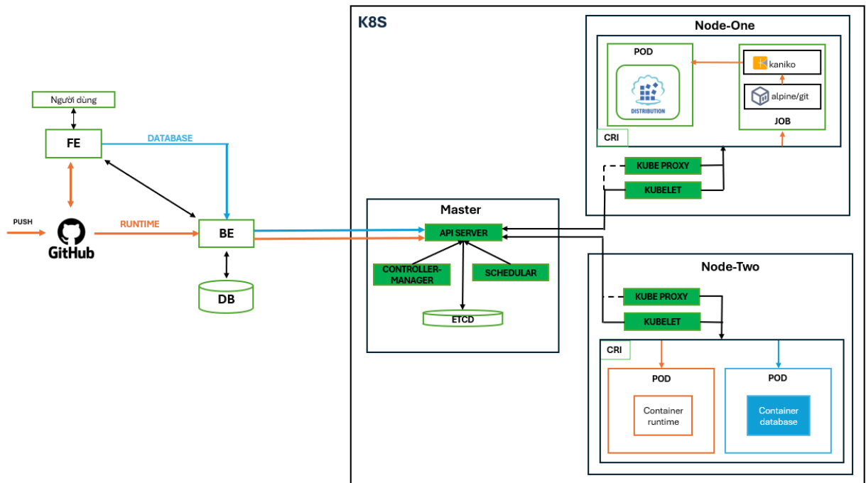
Hình 3.1 Kiến trúc hệ thống tổng quát
