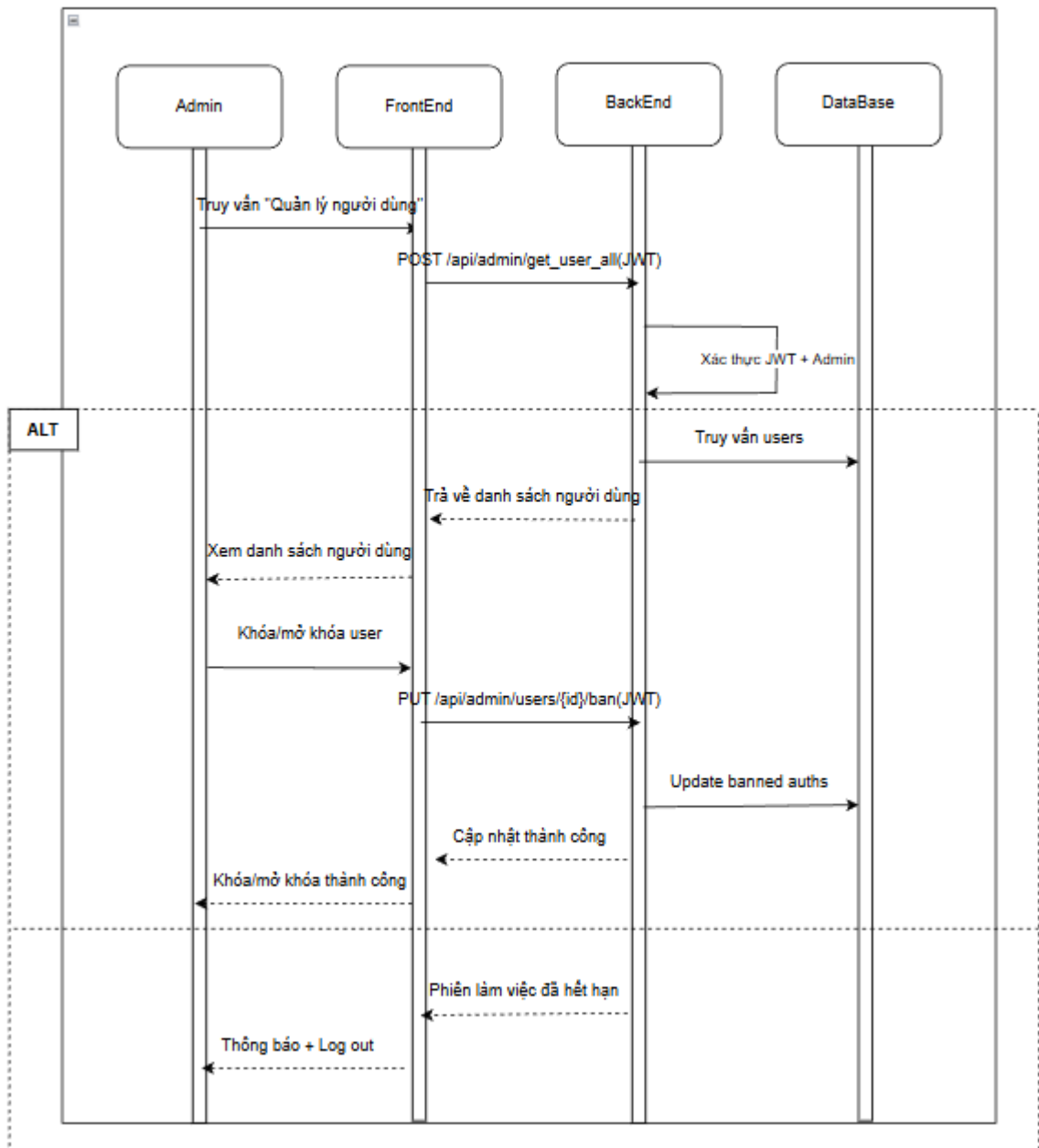
Hình 3.10 Quản lý người dùng
