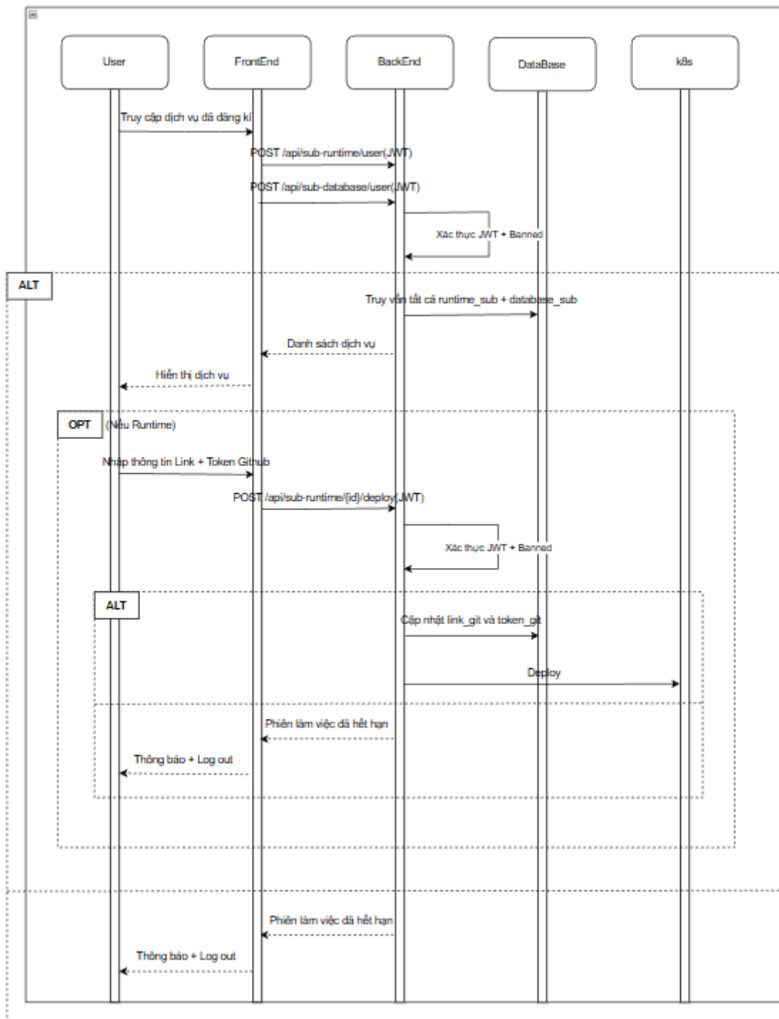
Hình 3.7 Biểu đồ tuần tự chức năng truy cập dịch vụ và chạy
