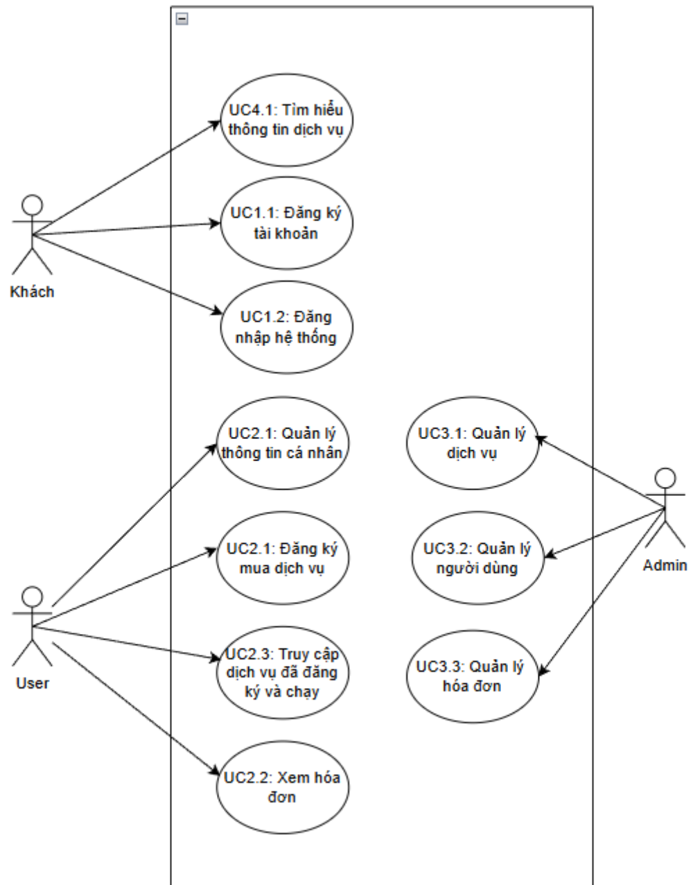
Hình 2.1. Sơ đồ Usecase tổng quát
