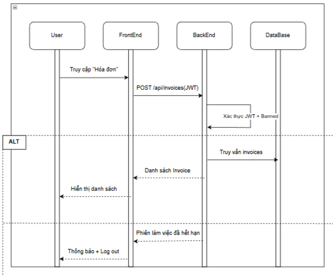
Hình 3.6 Biểu đồ tuần tự chức năng xem hóa đơn
