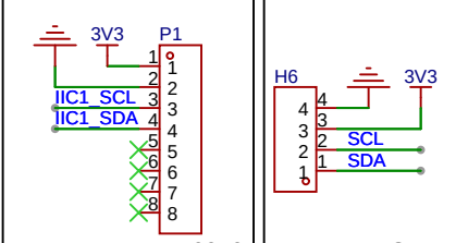
MPU6050
