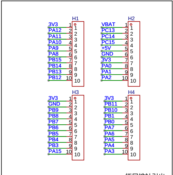
拓展排针引出
