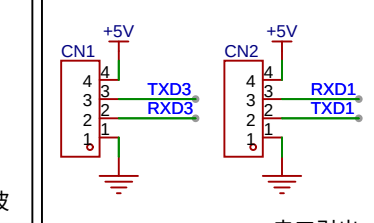
串口引出
