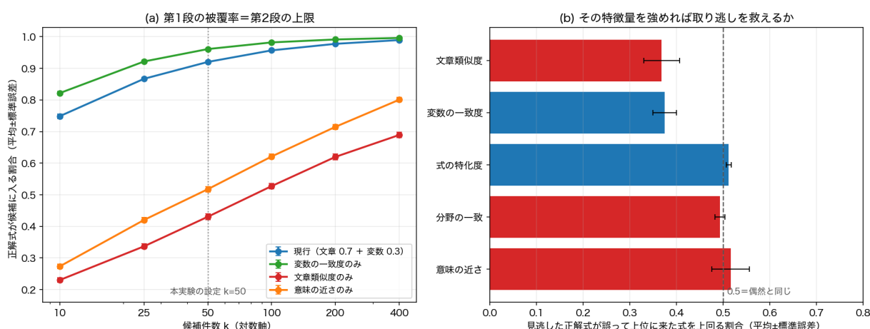
図 3 (a) 第 1 段の絞り込み方ごとの被覆率 (正解式が候補 k 件に入る割合。1,823 ケースの平均、誤差棒は標準誤差)。被覆率は第 2 段の Recall@ K の上限を与える。(b) 見逃した正解式が、代わりに上位へ来た誤りの式を各特徴量で上回る割合 (131 ケースの平均、誤差棒は標準誤差)。0.5 は偶然と同じで、その特徴量を強めても順位が戻らないことを意味する。
