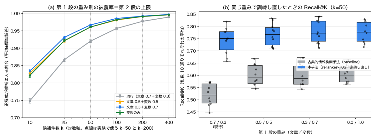
図2 第1段の重みを変える実験（設定A）。(a) 重み別の被覆率（1,823 ケースの平均 ± 標準誤差）。点線は実験で使う k = 50 と k = 200 。(b) 候補作り・訓練・評価を同じ重みで行なったときの \text{Recall}@K ( k = 50 。箱=乱数 10 通りの四分位、横線=中央値、点=各乱数の値)。被覆率の順序と最終精度の順序が一致し、文章 0.3 + 変数 0.7 が両方で最良になる。
