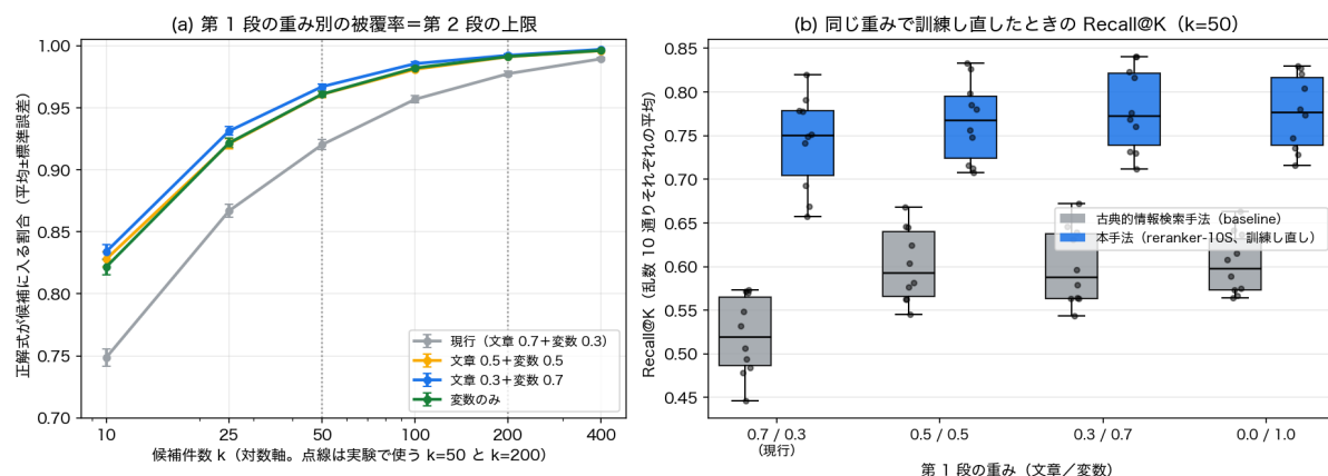
図 2 第 1 段の重みを変える実験（設定 A）。(a) 重み別の被覆率（1,823 ケースの平均 ± 標準誤差）。点線は実験で使う k = 50 と k = 200 。(b) 候補作り・訓練・評価を同じ重みで行なったときの Recall@K ( k = 50 。箱＝乱数 10 通りの四分位、横線＝中央値、点＝各乱数の値)。被覆率の順序と最終精度の順序が一致し、文章 0.3 + 変数 0.7 が両方で最良になる。
