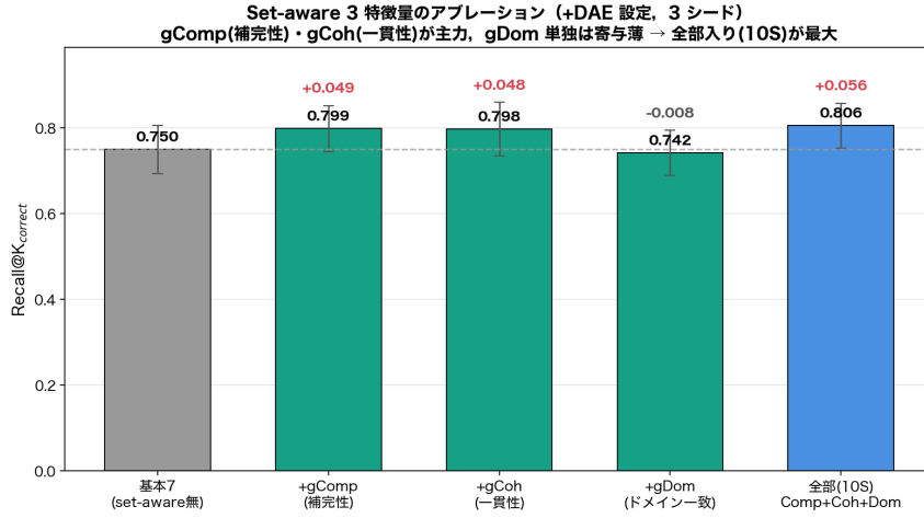
図7 Set-aware 3 特徴量のアブレーション (+DAE, 3 シード). gComp・gCoh が主力, gDom 単独は寄与薄, 3 つ全て (10S) が最良.
