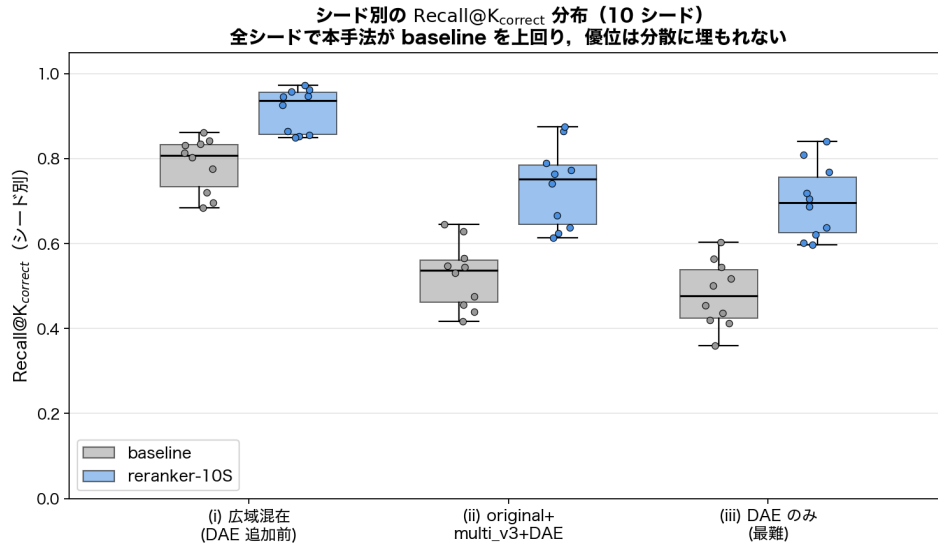
図8 3 設定での Recall@K correct のシード別分布 (10 シード, 点は各シード). 全シードで reranker-10S が baseline を上回る.
