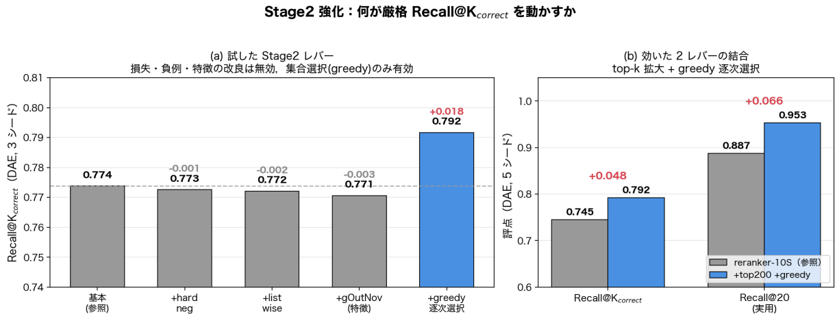
図 6 Stage2 強化で何が厳格 \text{Recall}@K_{\text{correct}} を動かすか. (a) 損失・負例・特徴の標準的改良は無効 ( \leq 0.006 , 3 シード), 集合選択を陽に行う greedy 逐次選択のみ +0.018. (b) 効いた 2 レバー (top- k 拡大 + greedy) の結合で \text{Recall}@K_{\text{correct}} +0.048 \cdot \text{Recall}@20 +0.066 (5 シード).
