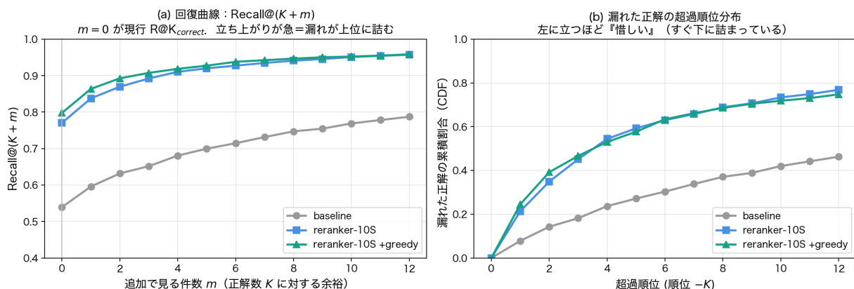
図 6 near-miss 分析 (DAE、候補 200 件予算)。(a) 回復曲線 \text{Recall}@ (K + m) ( m=0 が \text{Recall}@K_{correct} ) : reranker・greedy は急に立ち上がり K + 3 で \approx 0.9 。(b) 漏れた正解の超過順位 (順位 -K ) の累積分布：左に立つほど「惜しい」。
