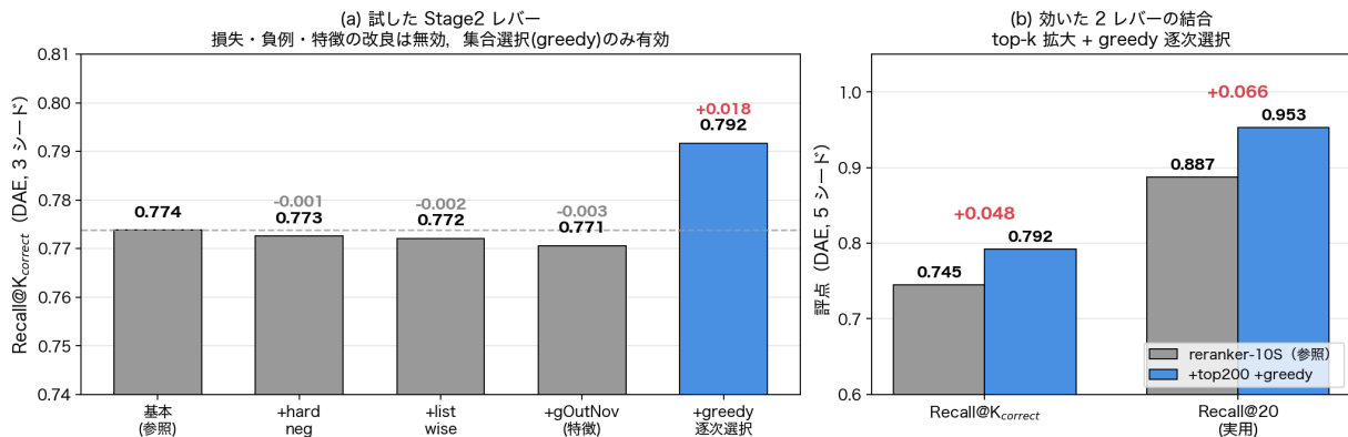
図 5 (a) 試した Stage 2 レバー：損失・負例・特徴の標準的改良は無効 ( \leq 0.006 )、集合選択 (greedy) のみ +0.018。(b) 効いた 2 レバー (top- k 拡大 + greedy) の結合で Recall@ K_{correct} +0.048・Recall@20 +0.066。
