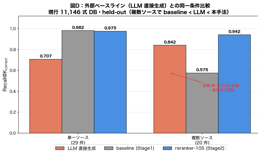
図 4 LLM 直接生成 vs baseline(Stage1) vs reranker-10S(Stage2) の同一条件比較 ( \text{Recall}@K_{\text{correct}} , 現行 11,146 式 DB). 複数ソースで baseline < LLM < 本手法.
