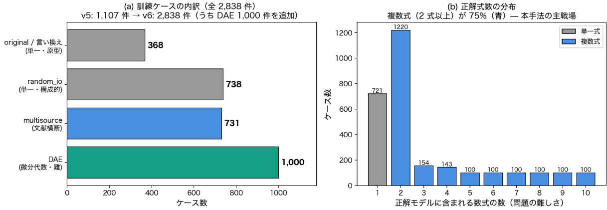
図 1 データセットの規模・内訳と難易度分布. (a) 訓練ケース 2,838 件の variant 別構成 (DAE 1,000 件を新規追加, 緑). (b) 正解式数の分布: 複数式 (2 式以上, 青) が全体の 74.6%.
