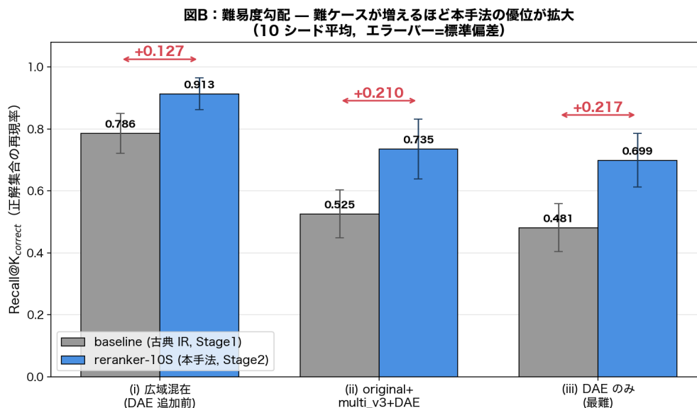
図2 難ケース比率の異なる3設定における \text{Recall}@K_{\text{correct}} (10 シード平均, エラーバー=標準偏差). 難ケースが増えるほど baseline は低下し, 本手法との差 (赤) が拡大する.
