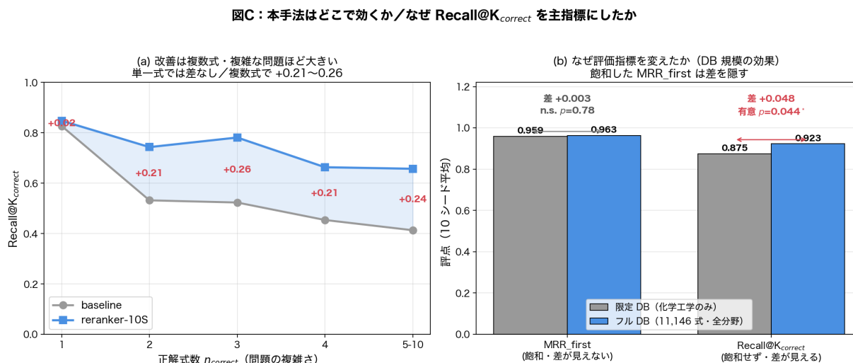
図3 (a) 正解式数別の \text{Recall}@K_{\text{correct}} : 改善は複数式・複雑な問題ほど大きい. (b) 仮説 B の再検定: 飽和した \text{MRR\_first} では差が見えないが, \text{Recall}@K_{\text{correct}} ではフル DB が有意に優位 ( p = 0.044 ).
