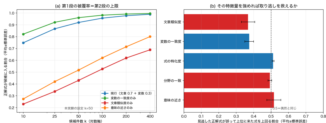
図3 (a) 第1段の絞り込み方ごとの被覆率（正解式が候補 k 件に入る割合。1,823 ケースの平均、誤差棒は標準誤差）。被覆率は第2段の \text{Recall}@K の上限を与える。(b) 上位 K 件に入らなかった正解式が、代わりに上位へ入った誤りの式を各特徴量で上回る割合（131 ケースの平均、誤差棒は標準誤差）。0.5 は偶然と同じで、その特徴量を強めても順位が戻らないことを意味する。
