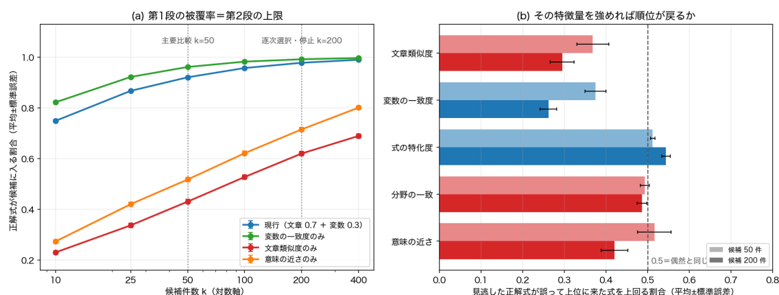
図 3 (a) 第 1 段の絞り込み方ごとの被覆率（正解式が候補 k 件に入る割合。1,823 ケースの平均、誤差棒は標準誤差）。被覆率は第 2 段の Recall@ K の上限を与える。(b) 上位 K 件に入らなかった正解式が、代わりに上位へ入った誤りの式を各特徴量で上回る組の割合（ケースごとに求めた割合の平均。候補 50 件は 131 ケース、200 件は 182 ケース。誤差棒は標準誤差）。0.5 は偶然と同じで、その特徴量を強めても順位が戻らないことを意味する。
