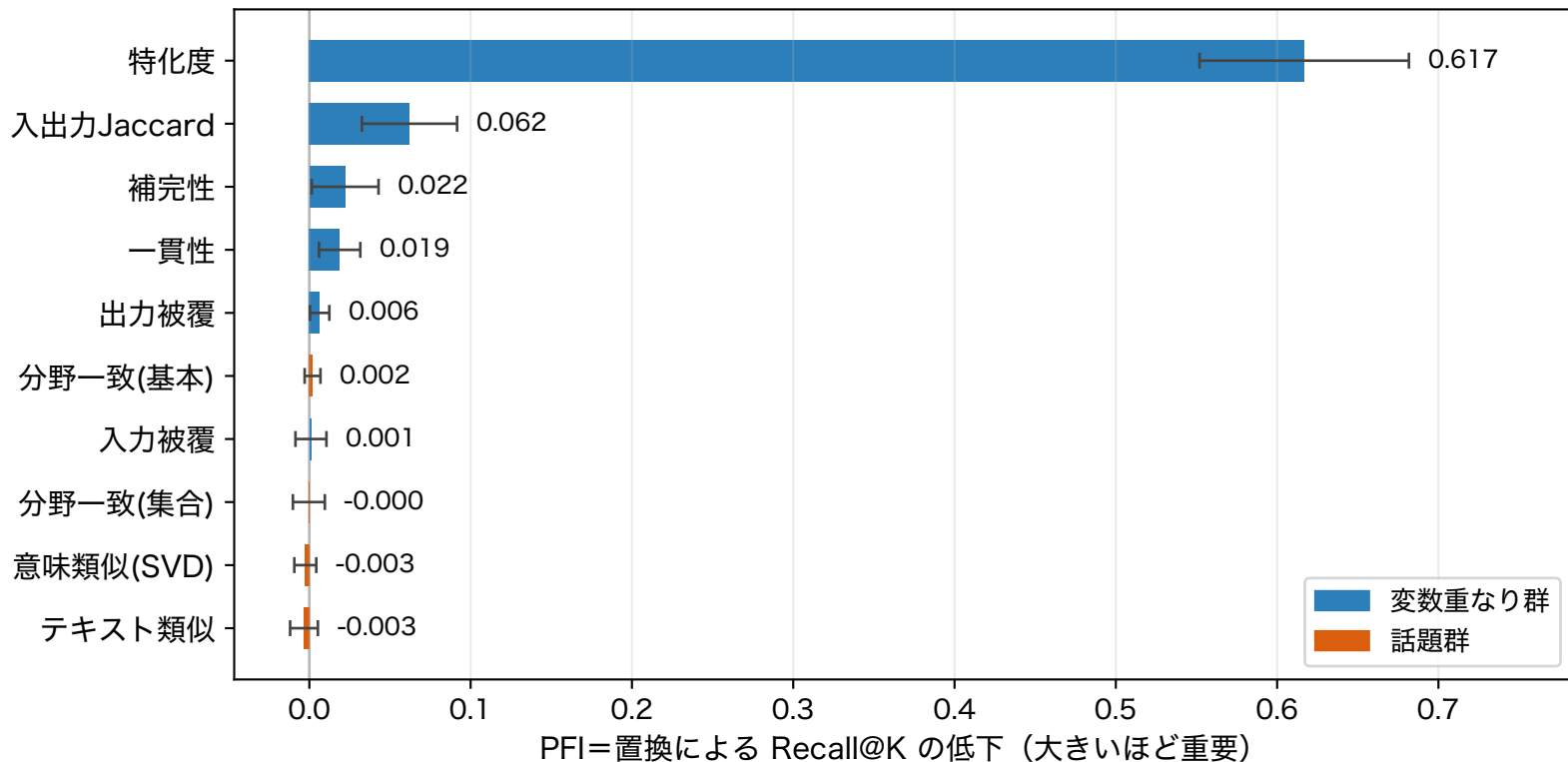
(a) 個別特徴量の重要度 (reranker-10S・10 seed)
