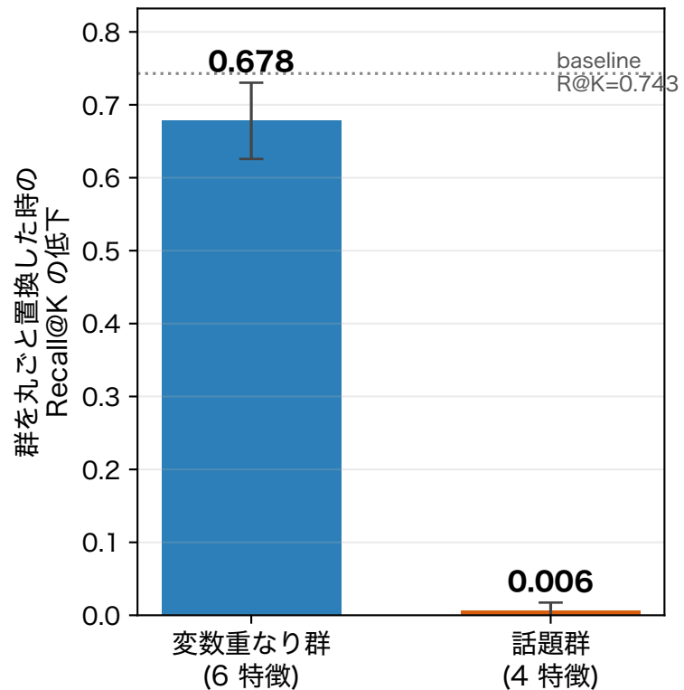
(b) 群ごとの重要度=機構
