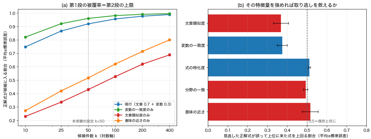
図2 (a) 第1段の絞り込み方ごとの被覆率（正解式が候補 k 件に入る割合。1,823 ケースの平均、誤差棒は標準誤差）。被覆率は第2段の Recall@ K の上限を与える。(b) 見逃した正解式が、代わりに上位へ来た誤りの式を各特徴量で上回る割合（131 ケースの平均、誤差棒は標準誤差）。0.5 は偶然と同じで、その特徴量を強めても順位が戻らないことを意味する。
