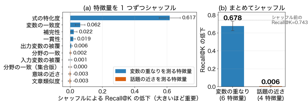
図 2 特徴量の値をケース内でシャッフルしたときの \text{Recall}@K の低下 (大きいほどモデルがその特徴量に頼っている)。誤差棒は乱数 10 通りの標準偏差。(b) の点線はシャッフル前の \text{Recall}@K = 0.743 。
