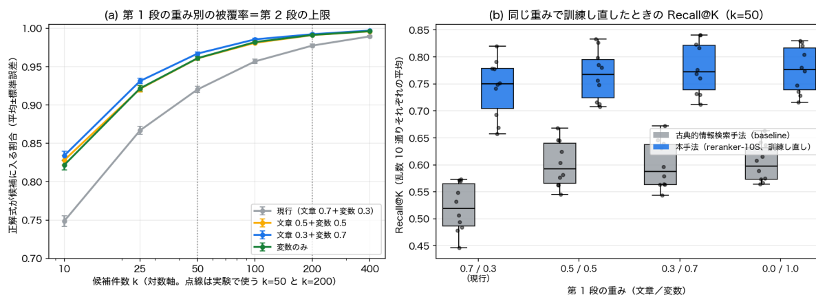
図 2 第 1 段の重みを変える実験（設定 A）。(a) 重み別の被覆率（1,823 ケースの平均 ± 標準偏差）。点線は実験で使う k = 50 と k = 200 。(b) 候補作り・訓練・評価を同じ重みで行なったときの \text{Recall}@K ( k = 50 。箱 = 乱数 10 通りの四分位、横線 = 中央値、点 = 各乱数の値)。被覆率の順序と最終精度の順序が一致し、文章 0.3 + 変数 0.7 が両方で最良になる。
