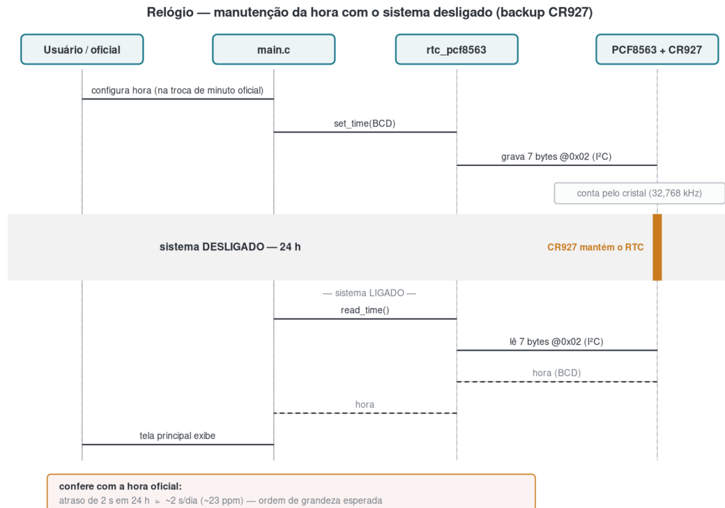
Figura 37 – Sequência do ensaio de manutenção da hora com o sistema desligado
