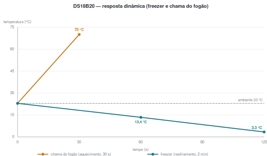
Figura 31 – Resposta do DS18B20 aos transientes de resfriamento e aquecimento
