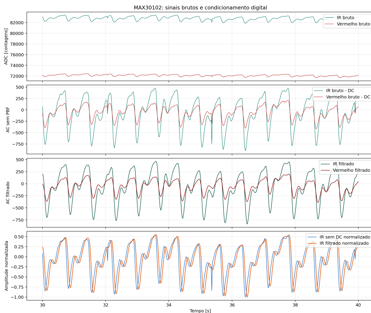
Figura 29 – Ampliação de 30 a 40 s e comparação normalizada do canal infravermelho
