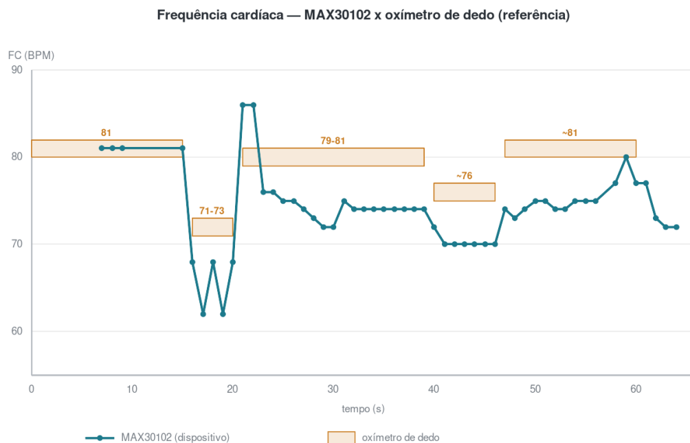
Figura 30 – Frequência cardíaca indicada pelo MAX30102 e faixa observada no oxímetro
