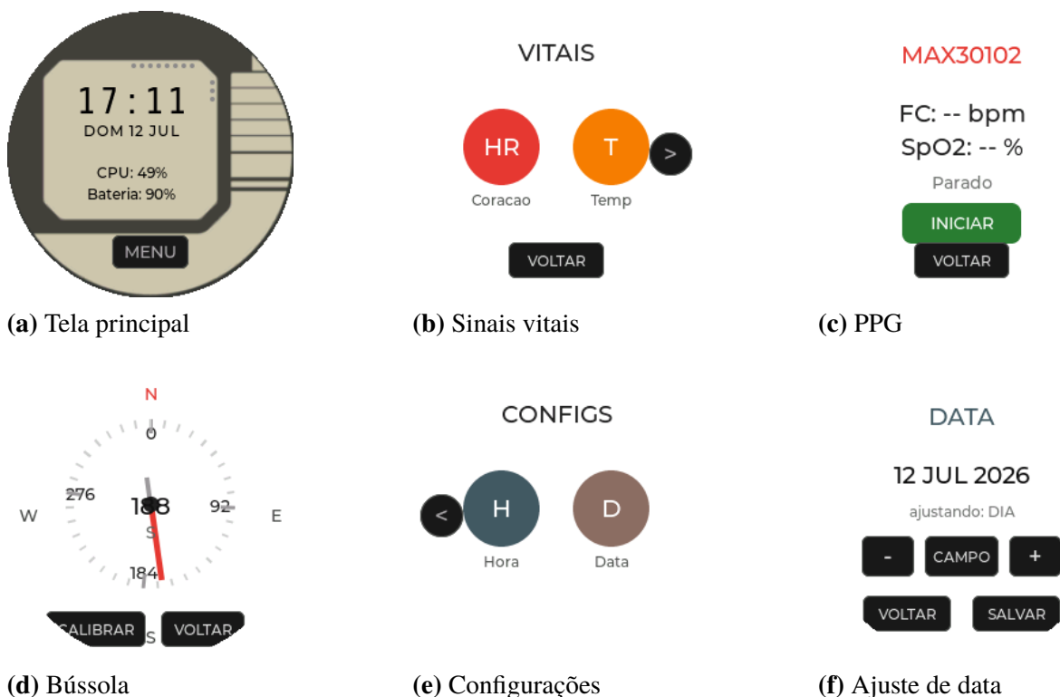
Figura 36 – Capturas da interface executável da plataforma
