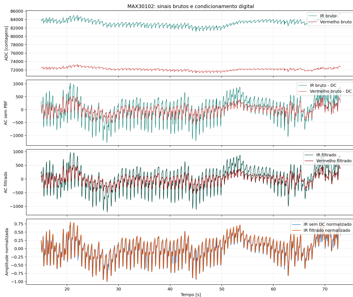
Figura 28 – Canais PPG brutos, sem componente DC e filtrados no intervalo estabilizado de 15 a 73 s
