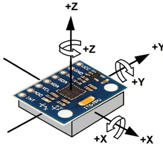
(b) Ejes de sensibilidad triaxial ( +X , +Y , +Z )
