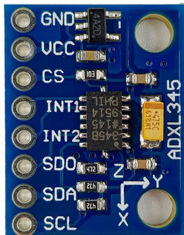
(a) Módulo sensor acelerometro ADXL345
