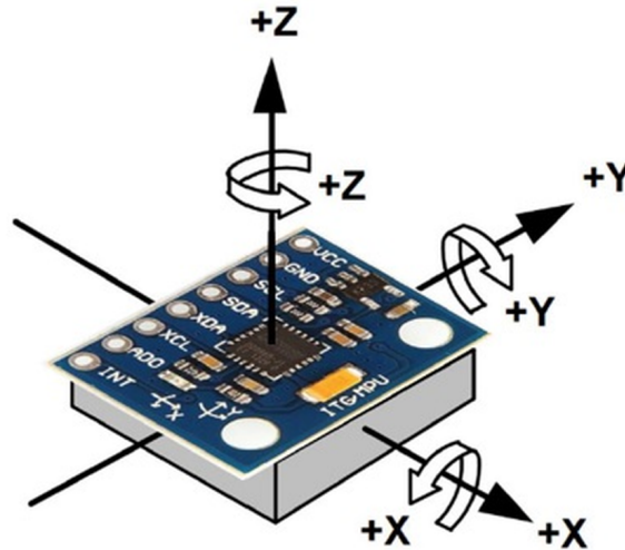
(b) Ejes de sensibilidad triaxial (+X, +Y, +Z)
