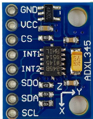
(a) Módulo sensor acelerómetro ADXL345
