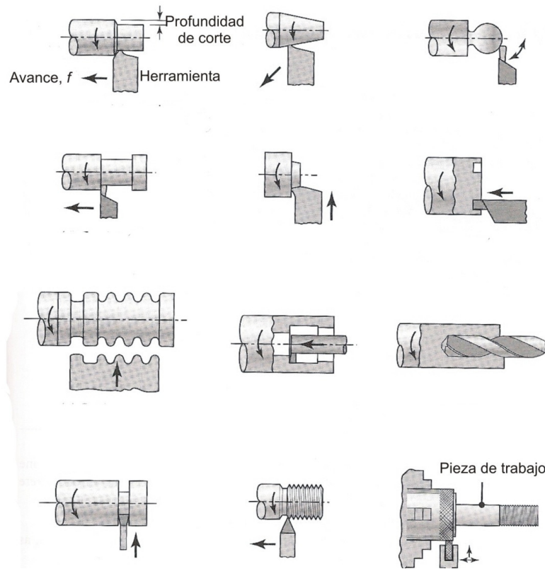
Figura 2 Operaciones fundamentales de mecanizado por arranque de viruta en torno CNC
