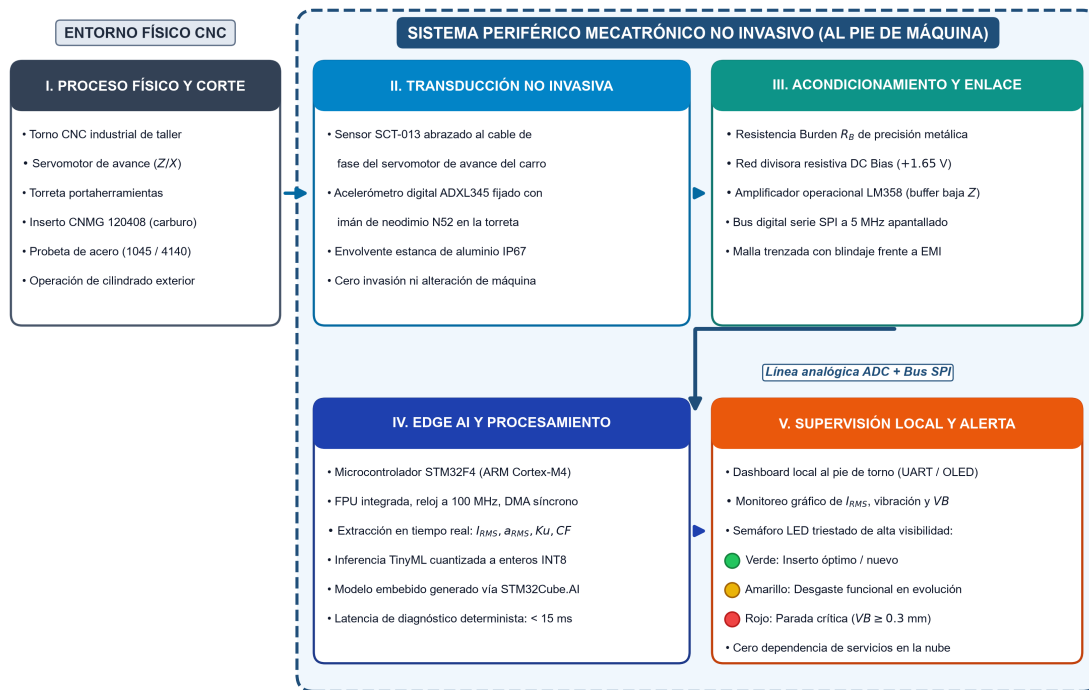
Figura A.1 Diagrama de bloques funcional general de la arquitectura mecatrónica periférica para monitoreo no invasivo en tornos CNC
