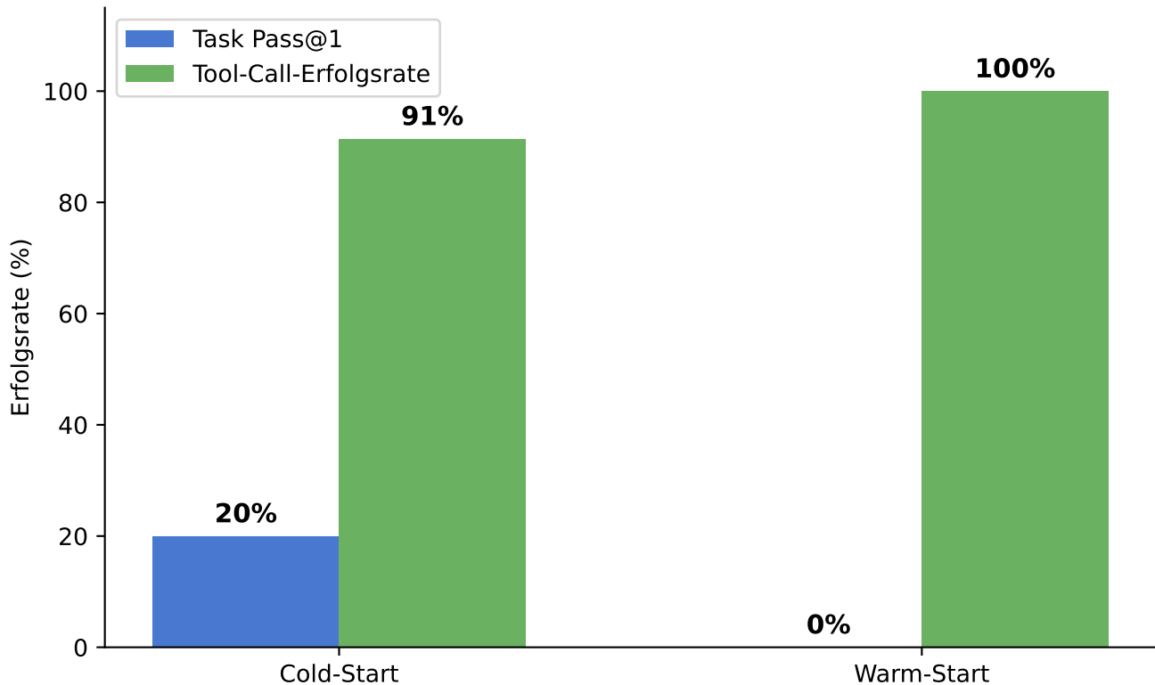
L5 DB-Benchmark: Skill-Qualität vs Task-Erfolg
