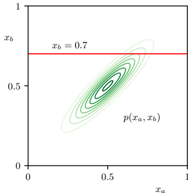
Abbildung: Links: Zweidimensionale Normalverteilung. Rechts: Randverteilung für x_a in blau. Siehe [2], Seite 82.
