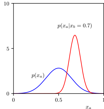
Abbildung: Links: Zweidimensionale Normalverteilung. Rechts: Randverteilung für x_a in blau. Siehe [2], Seite 82.
