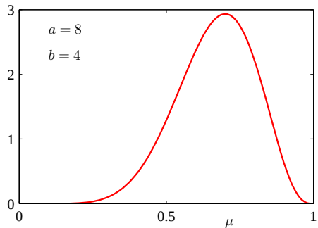
Abbildung: Beta-Verteilungen für einige Parameter a , b . Siehe Bishop2006 , Seite 72.
