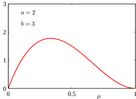
Abbildung: Beta-Verteilungen für einige Parameter a , b . Siehe Bishop2006 , Seite 72.
