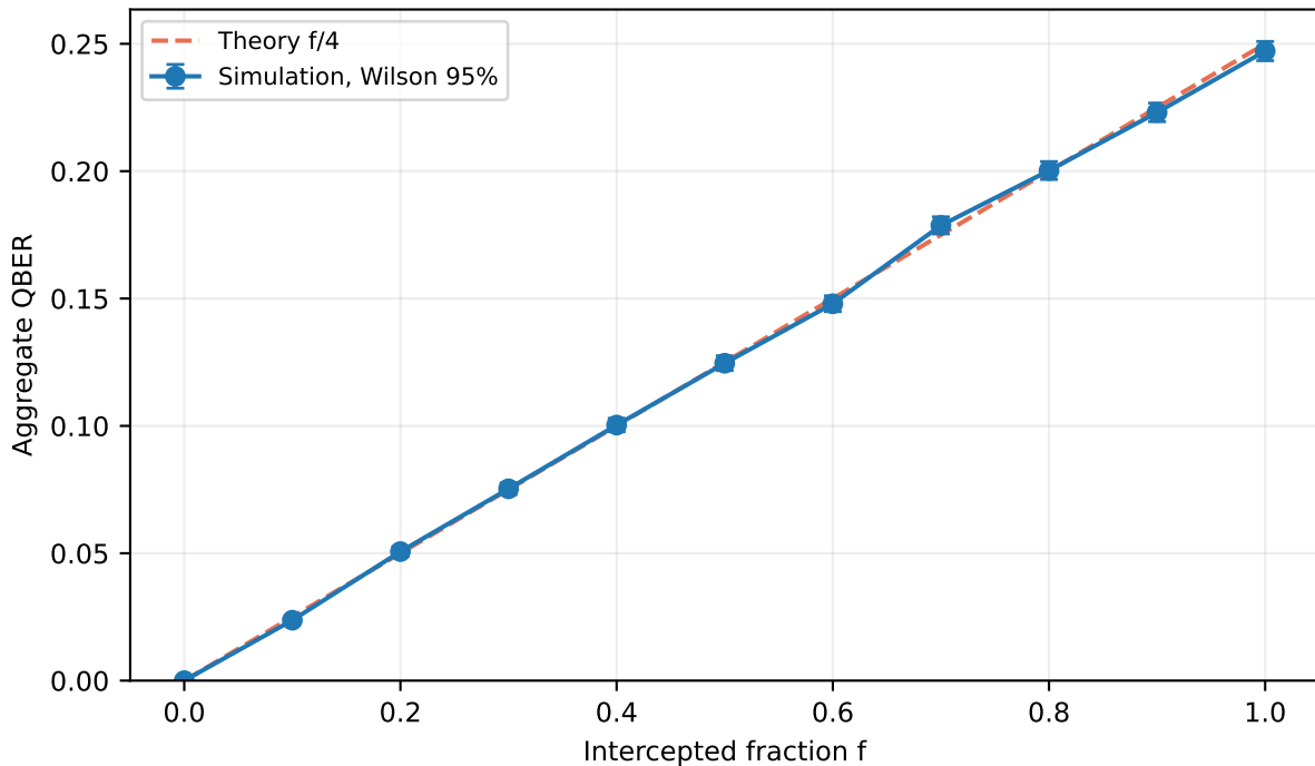
E3 intercept-resend QBER
