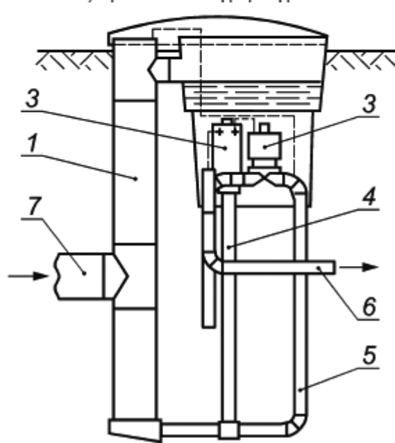
б) Отдельно стоящий приемный колодец
