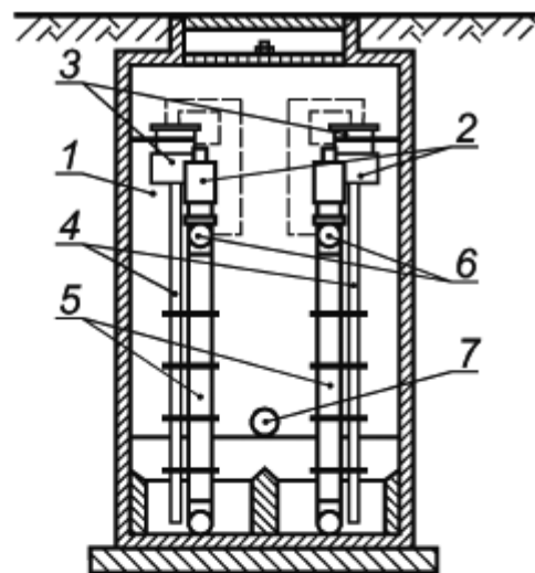
б) Приемный колодец на два клапана
