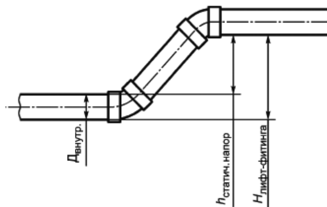
Рисунок И.2 - Схема расчета лифт-фитингов
