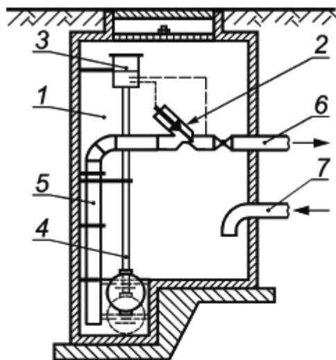
а) Клапан внутри приемного колодца
