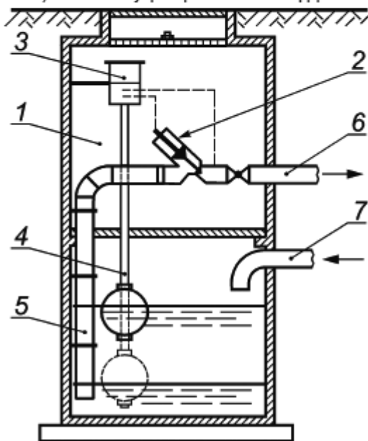
а) Клапан внутри приемного колодца
