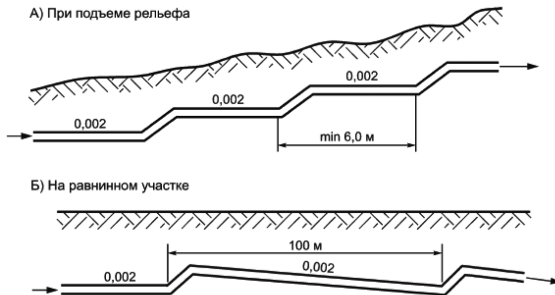
Рисунок И.1 - Принципы построения профилей сетей вакуумной канализации
