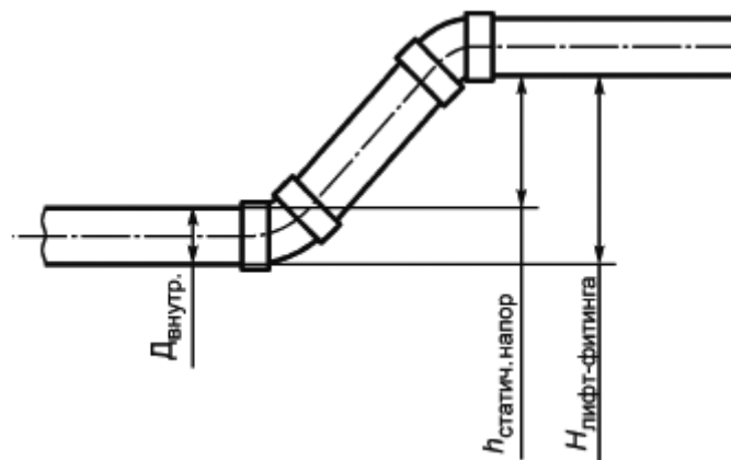
Рисунок И.2 - Схема расчета лифт-фитингов
