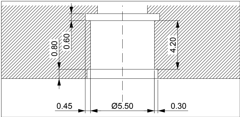
Detalle B Escala 5:1
