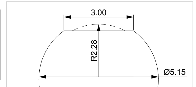
DETALLE C ESCALA 10:1
