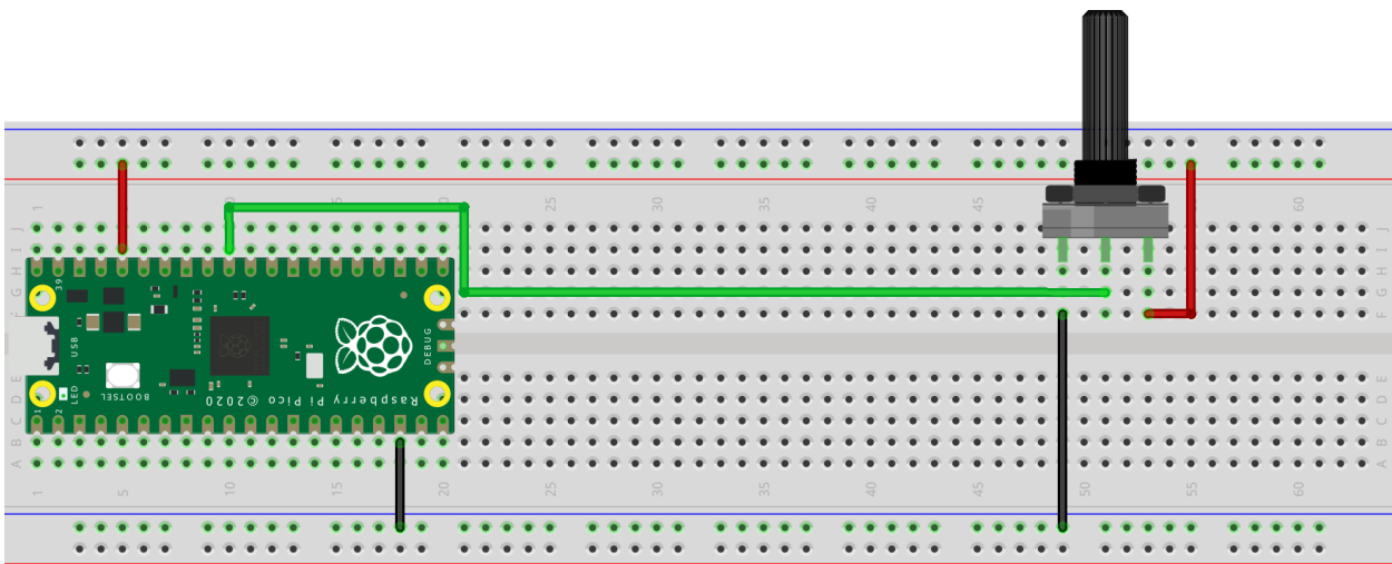
Bild 1: Schaltplan Potentiometeranschluss
