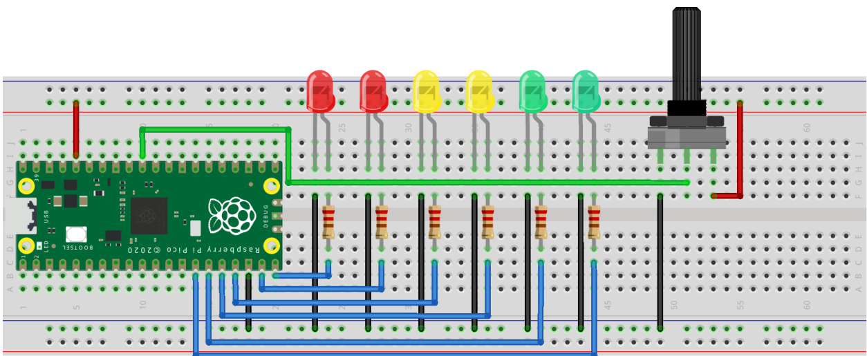
Bild 2: LEDs mit Potentiometer steuern
