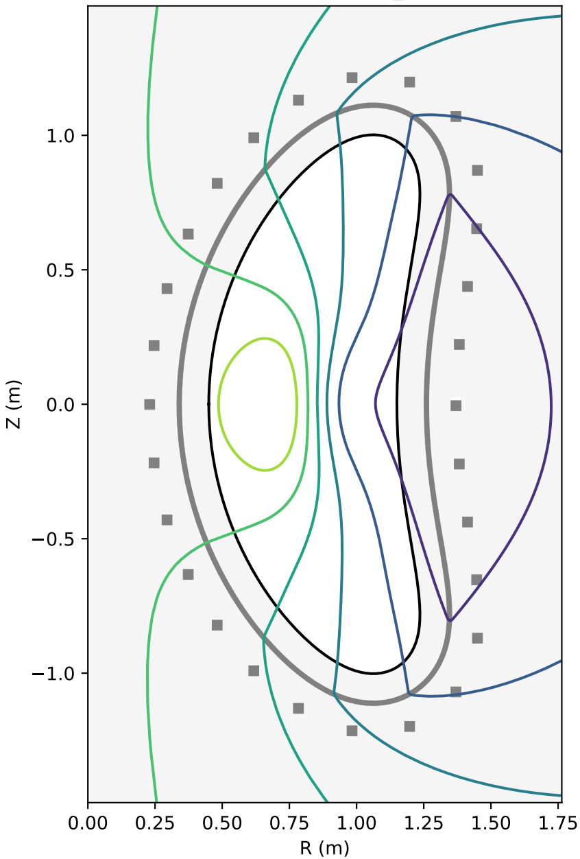
Unstable eigenmode \gamma\tau_w = -0.568
