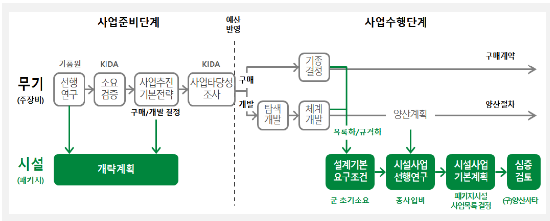
<그림 1> 주장비와 연계된 패키지시설사업 획득 절차
