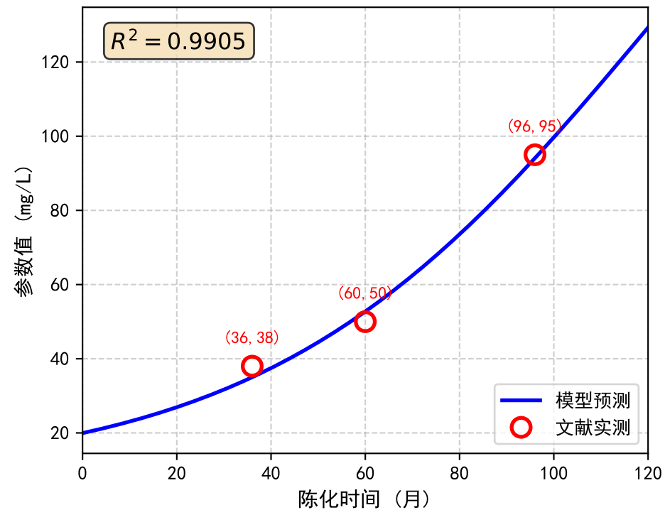
川芎嗪(TMP)陈化曲线
