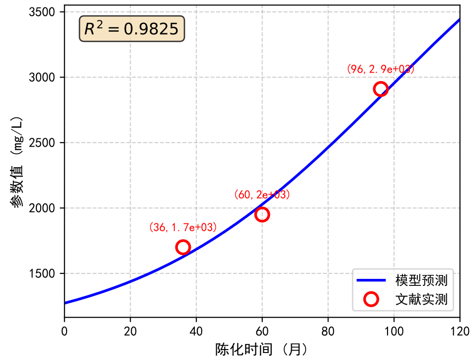
乙酸乙酯陈化曲线
