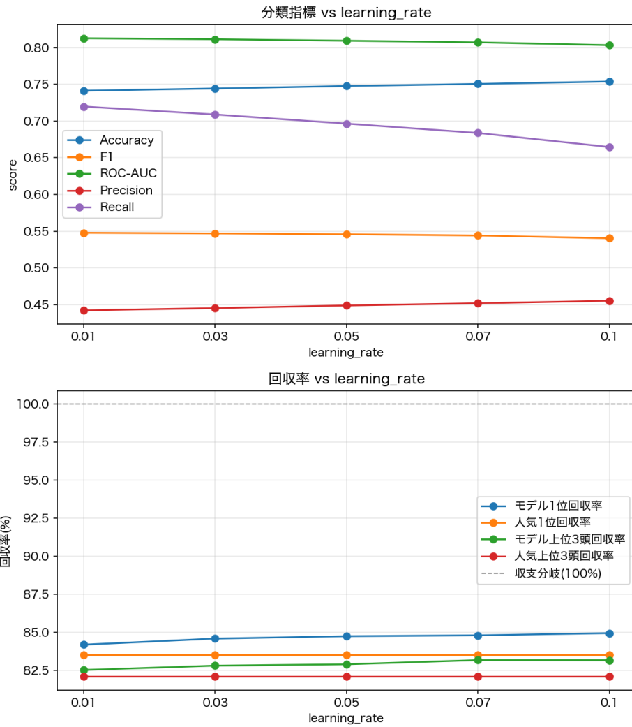
図2 分類指標・回収率 vs learning_rate (max_depth=7、採用)
