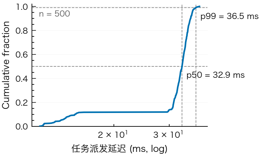
图 5.1 任务派发延迟经验累积分布 (n=500)
