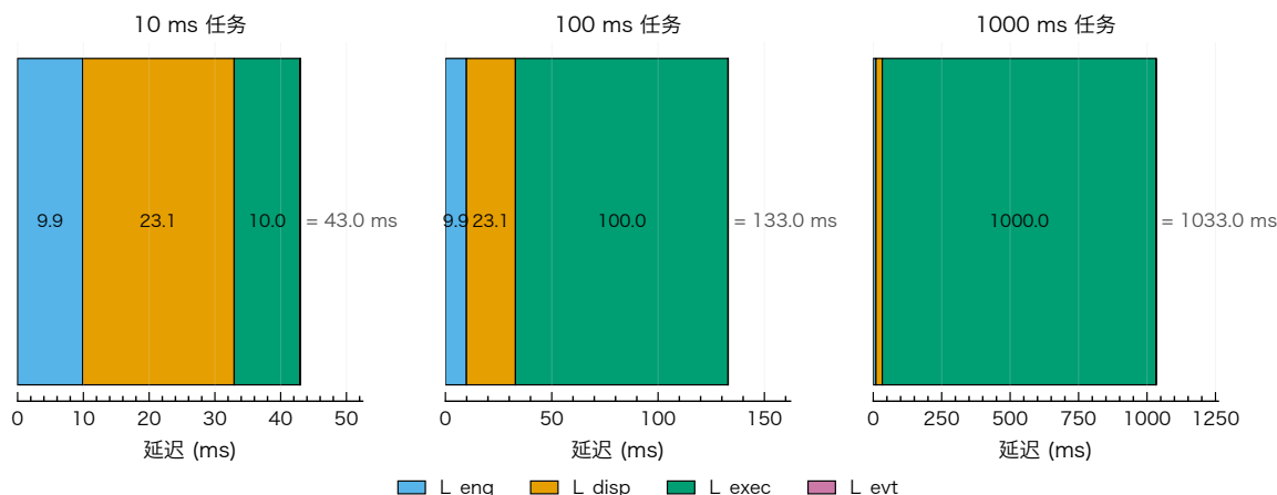
图 5.6 端到端延迟分解示意（公式 (2-3) 各分量；其中 L_{enq} 与 L_{disp} 为对 task_dispatch p50 的 3:7 估算拆分，非独立 profiler 实测）
