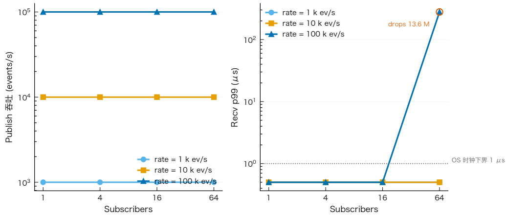
图 5.5 事件总线 publish 吞吐与丢帧率随订阅者数变化（右图 p99 为 log 轴；p99 < 1 μs 的样本受 macOS SystemTime ns→us 截断分辨率限制，统一显示为 0.5 μs）
