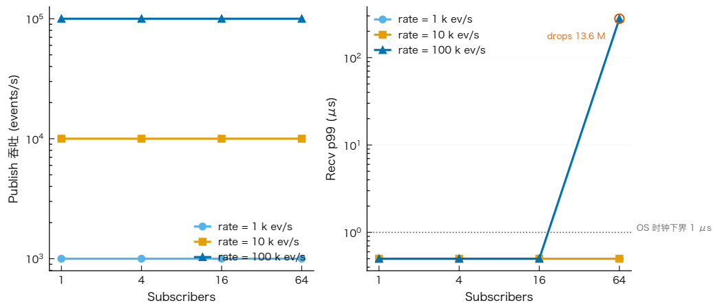
图 5.5 事件总线 publish 吞吐与丢帧率随订阅者数变化（右图 p99 为 log 轴；p99 < 1 μs 的样本受 macOS SystemTime ns 截断分辨率限制，统一显示为 0.5 μs）
