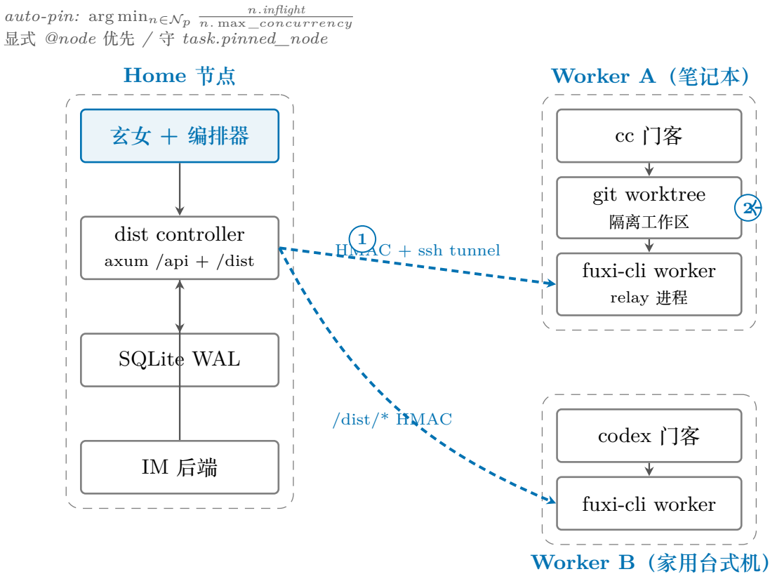
图 2.4 跨节点部署架构 (home 节点 + worker 节点 + 项目 host_nodes 路由)
