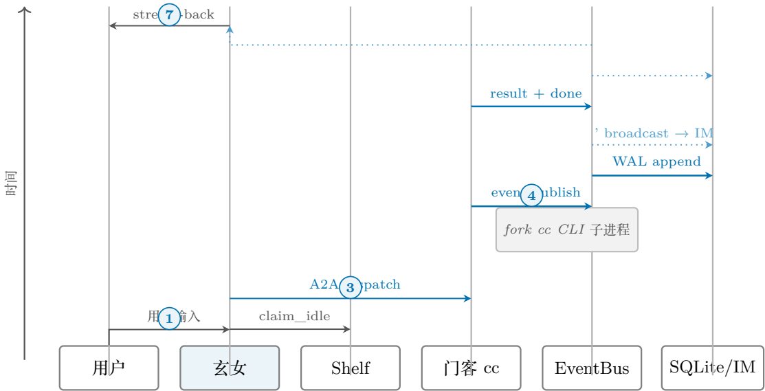
图 2.3 用户请求的端到端数据流（玄女接收 → dispatch → 门客 → EventBus → 多端扇出）
