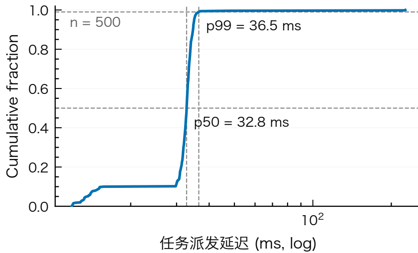
图 5.6 任务派发延迟经验累积分布 (n=500)
