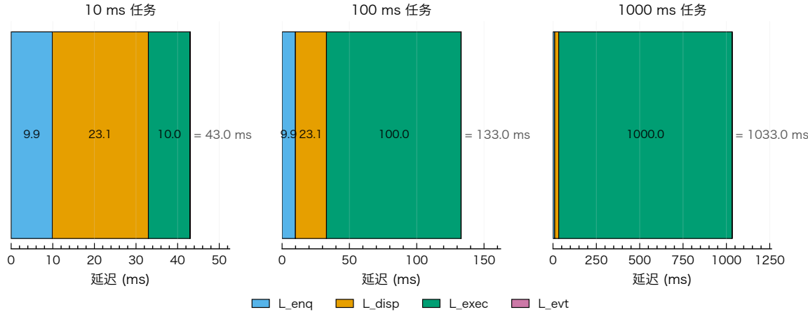
图 5.11 端到端延迟分解（公式 (2-1) 各分量实测）
