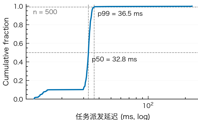
图 5.6 任务派发延迟经验累积分布 (n=500)
