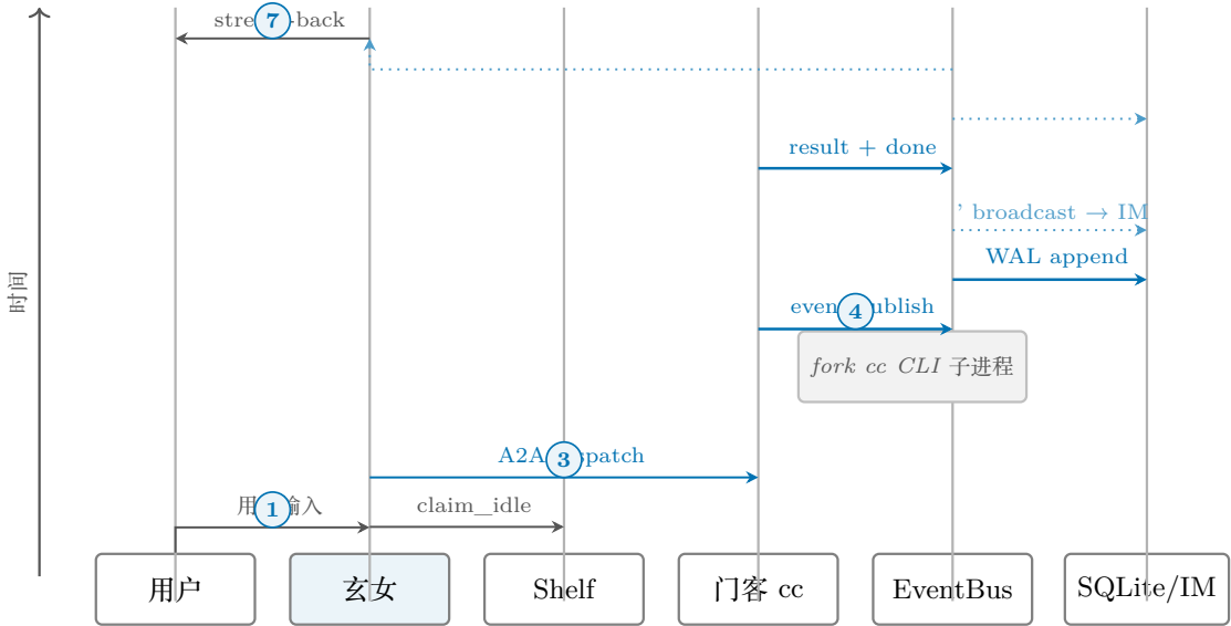
图 2.3 用户请求的端到端数据流（玄女接收 → dispatch → 门客 → EventBus → 多端扇出）
