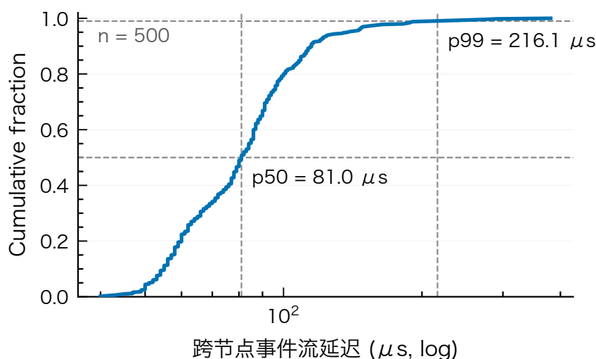
图 5.7 跨节点事件流延迟经验累积分布 (n=500)
