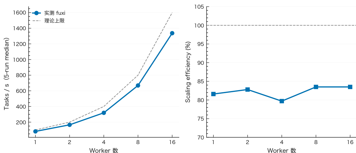
图 5.8 Worker 数对吞吐量（左）与扩展效率（右）的影响
