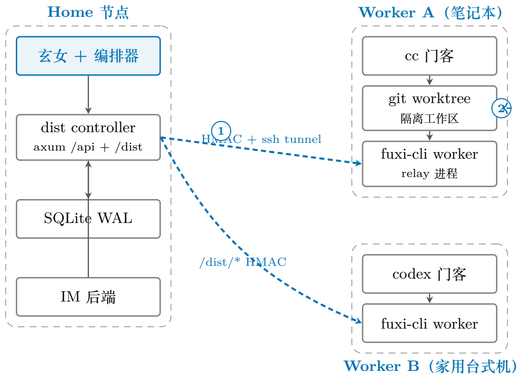
图 2.4 跨节点部署架构 (home 节点 + worker 节点 + 项目 host_nodes 路由)
