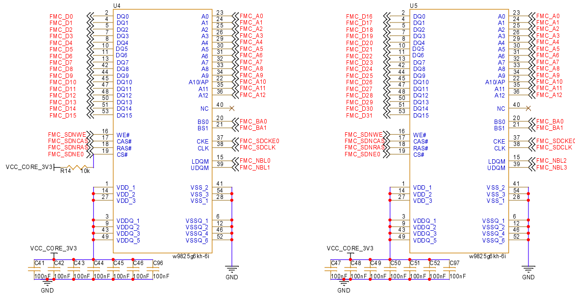
两片16位SDRAM组成32位
