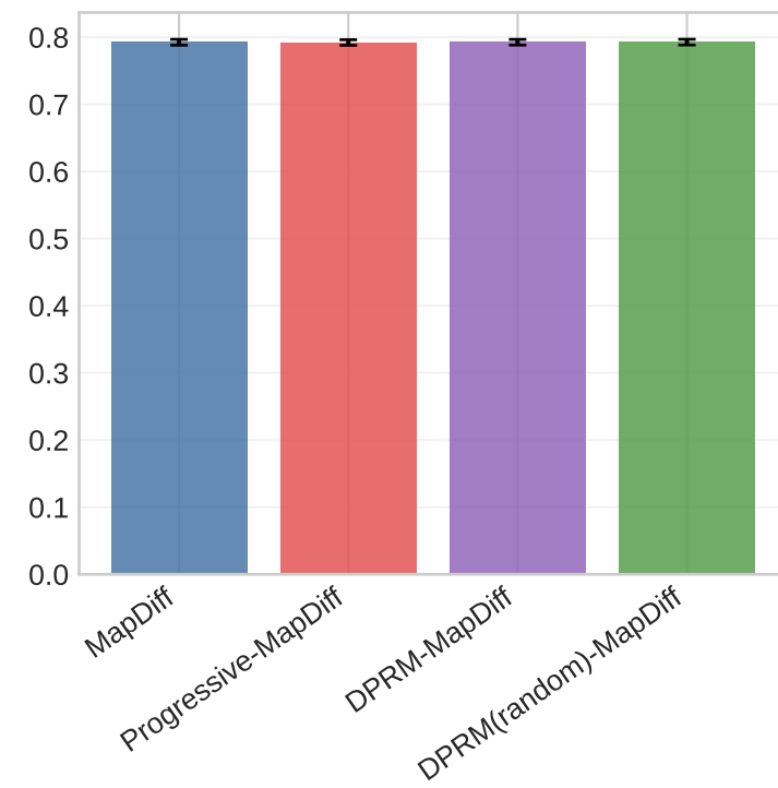
BLOSUM45 NSSR
