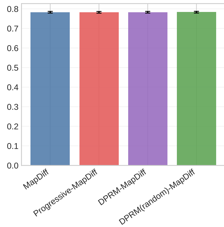
BLOSUM80 NSSR
