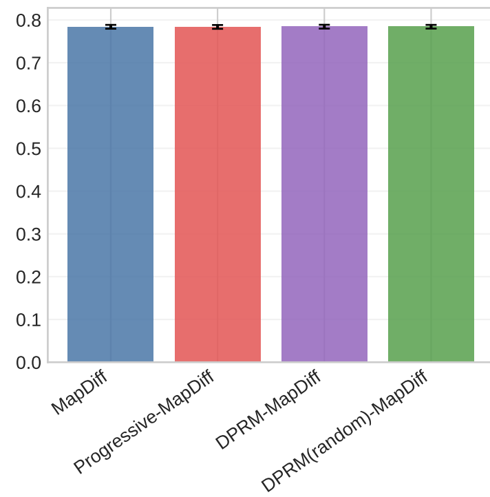
BLOSUM62 NSSR
