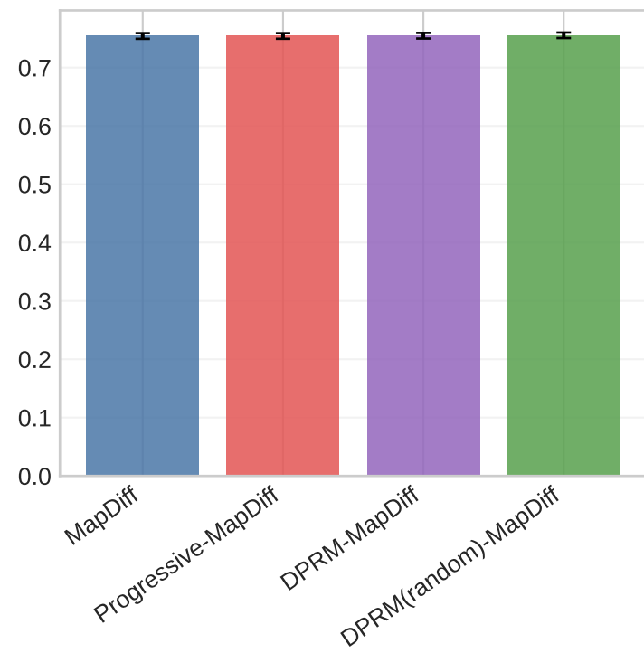
BLOSUM90 NSSR
