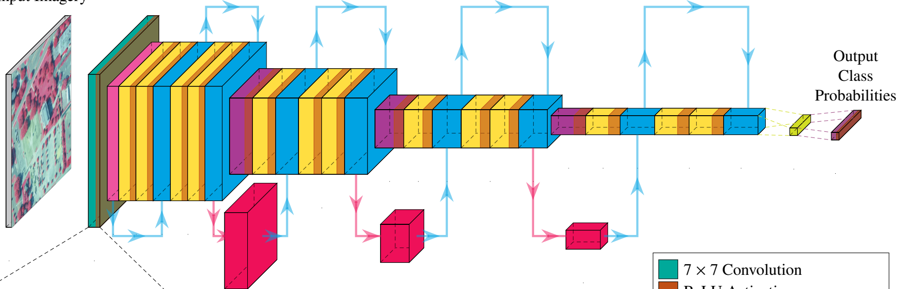
Input Imagery
